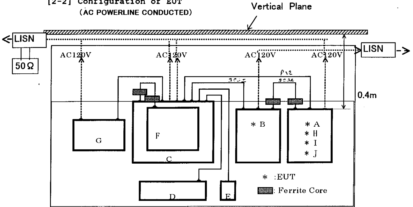
EUT Table : 2.1(W) × 1.0(D) × 0.8(H) (M)
