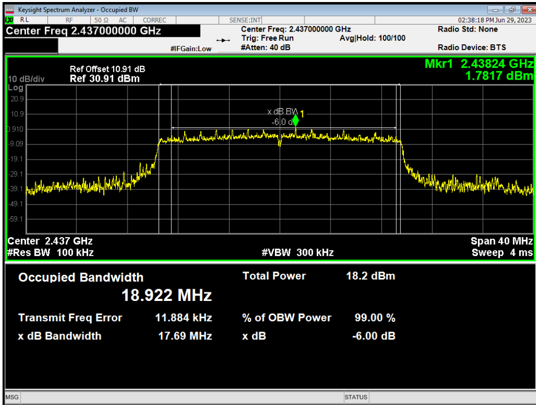
-6dB Bandwidth 802.11ax(HE20) 2437MHz
