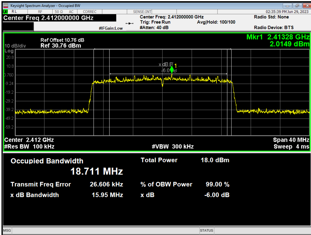
-6dB Bandwidth 802.11ax(HE20) 2412MHz
