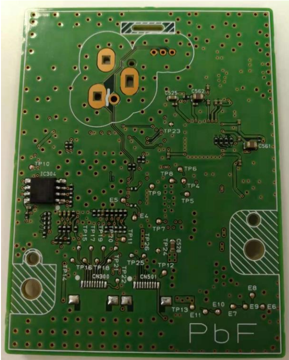
FACE PLATE_A SIDE
