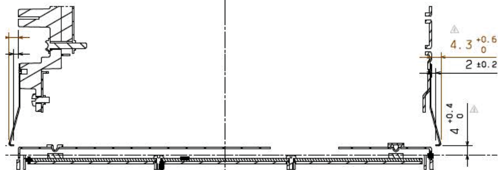
Section cut D-D Scale: 1:1
