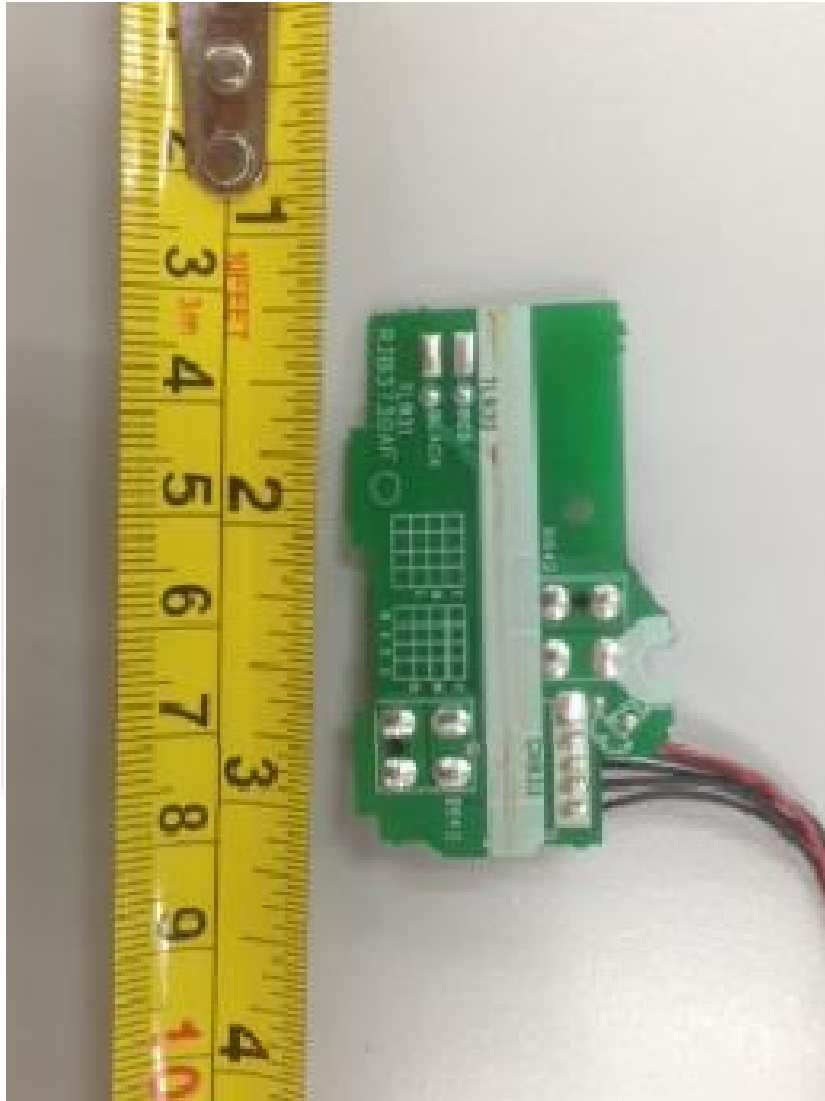
Door Switch PCB Trace Side
