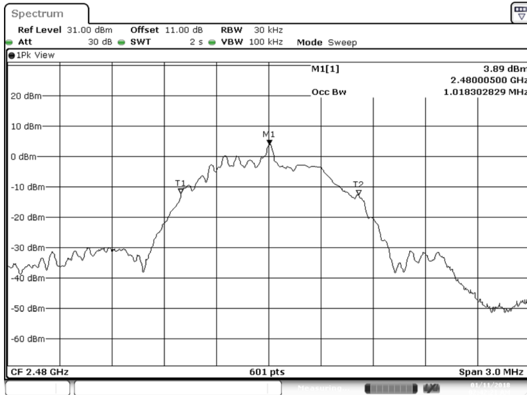
Plot3 99 Percent BW BLE 2480 MHz
