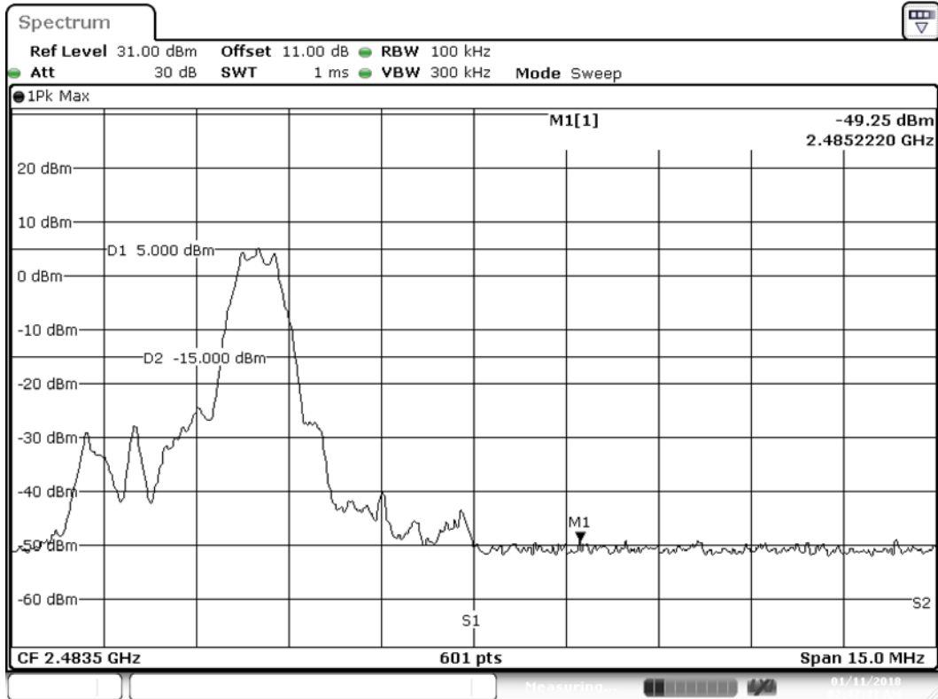
Plot1 Upper Band Edge BLE Peak 2480 MHz
