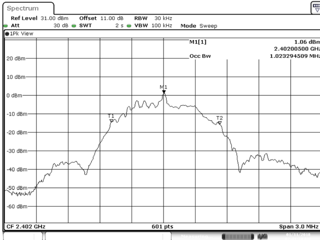
Plot1 99 Percent BW BLE 2402 MHz
