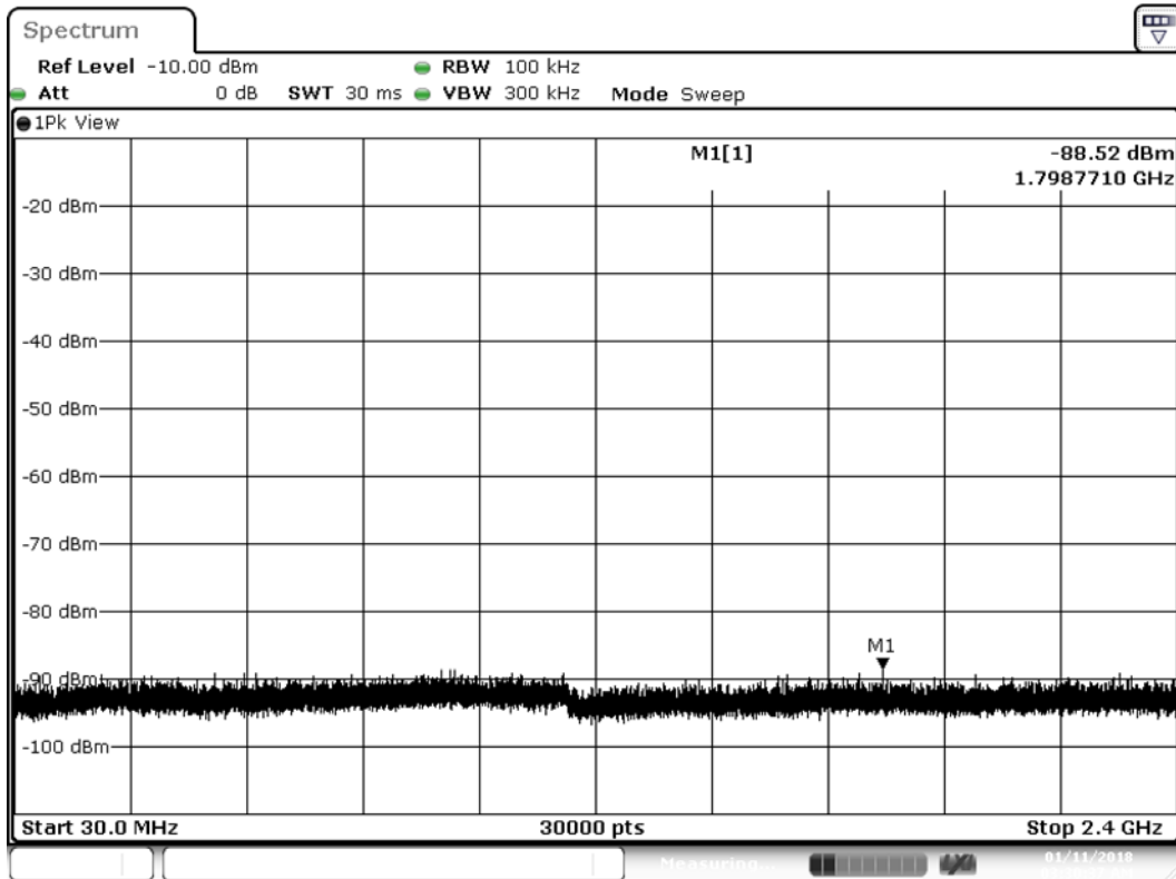
Plot1 BLE 2480 MHz Peak Band 1
