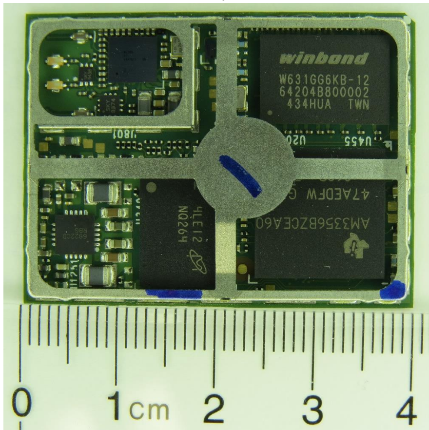
Module component site
