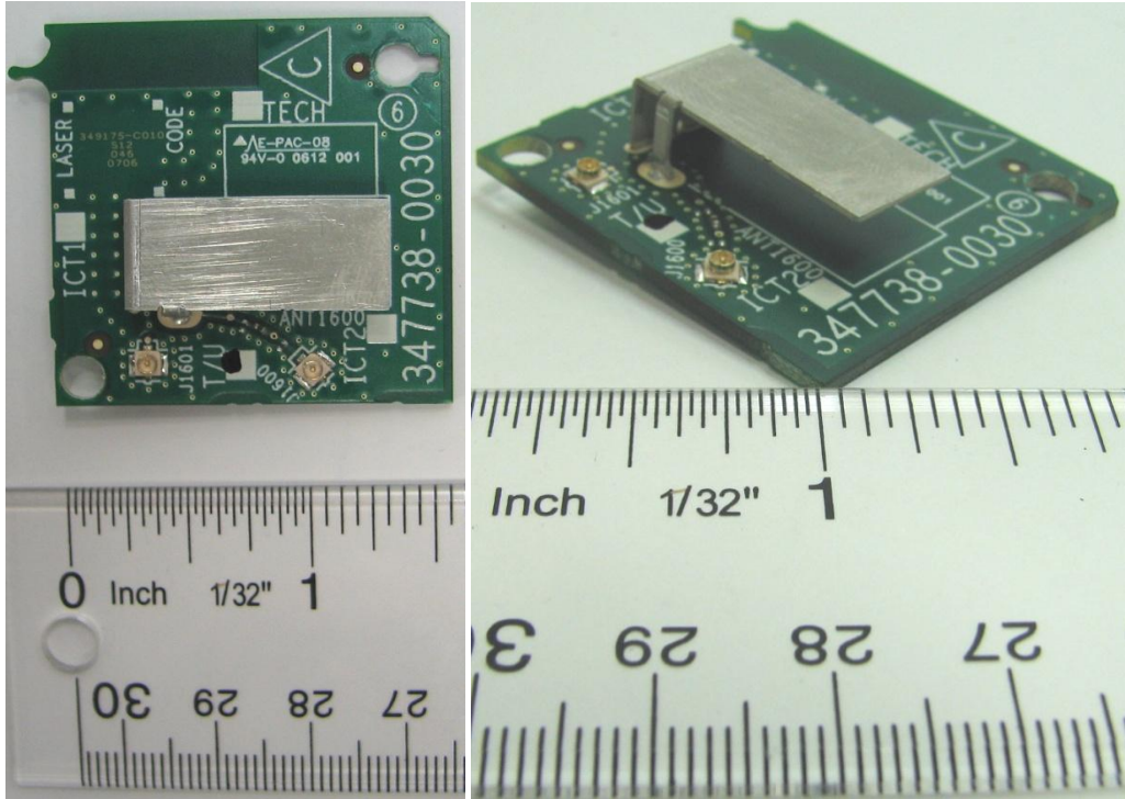
PIFA antenna
