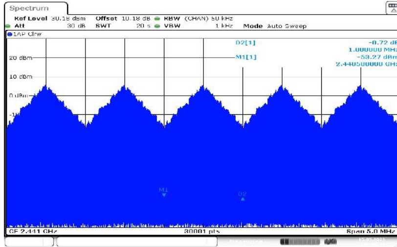
DH5 hopping
