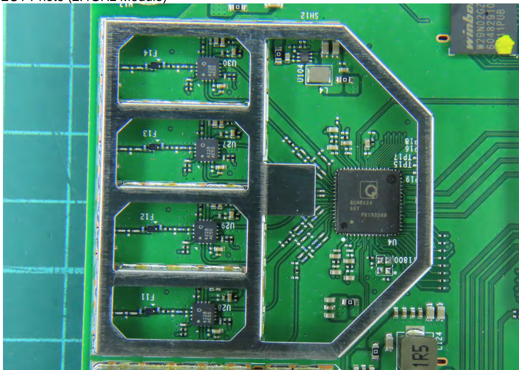
(10) EUT Photo (2.4GHz Module)
