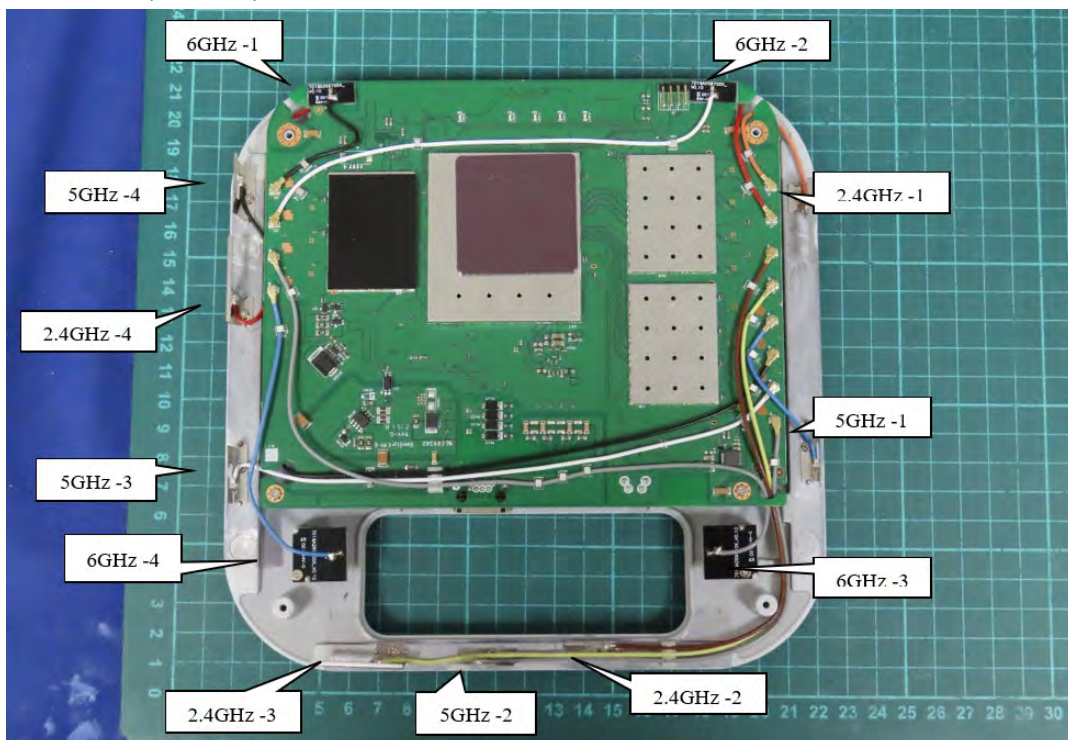
(2) EUT Photo (Antenna)
