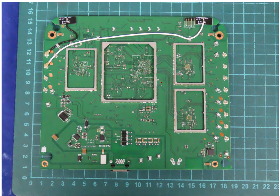
(6) EUT Photo
