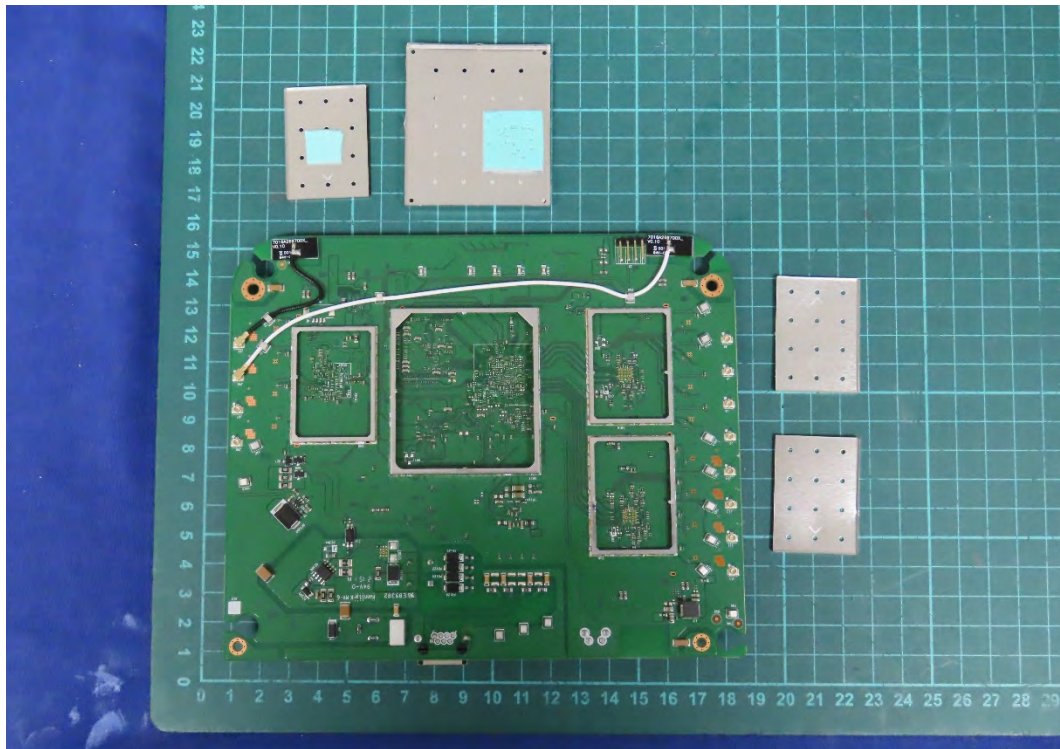
(6) EUT Photo
