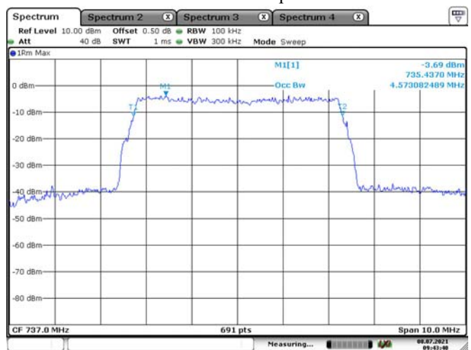
WCDMA-Output
