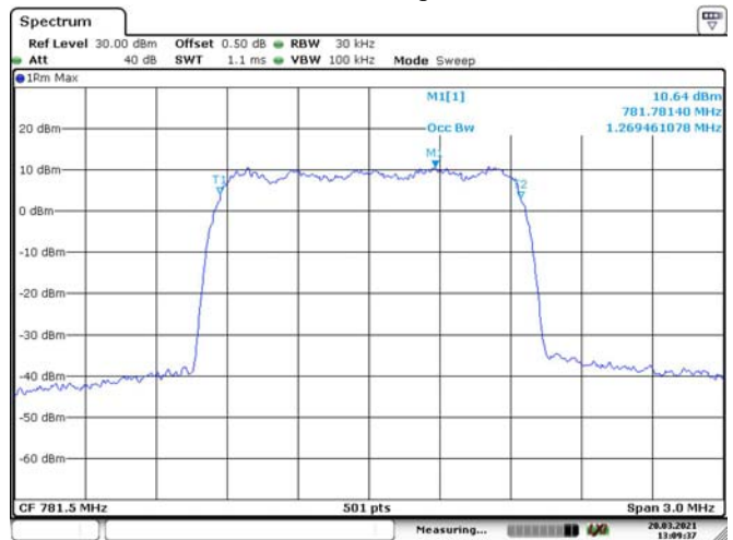
CDMA-Output
