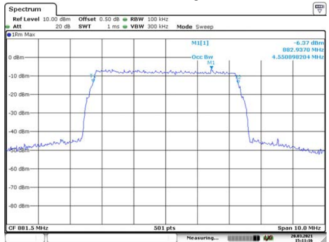
WCDMA-Output
