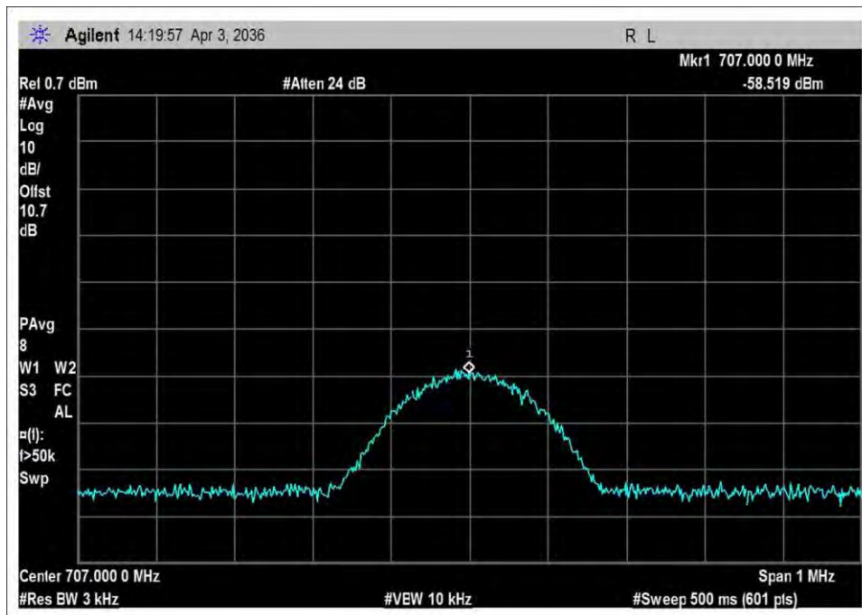
UL_698-716_input_GSM
