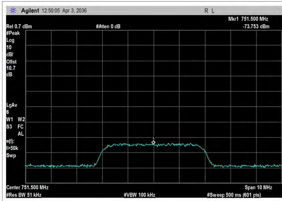
DL_746-757_input_WCDMA
