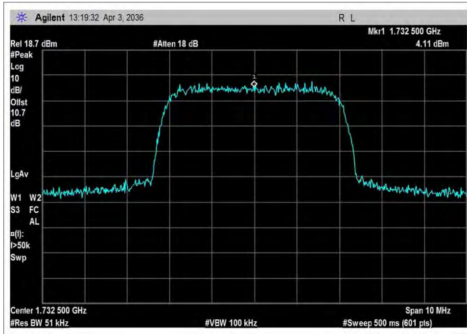
UL_1710-1755_output_WCDMA
