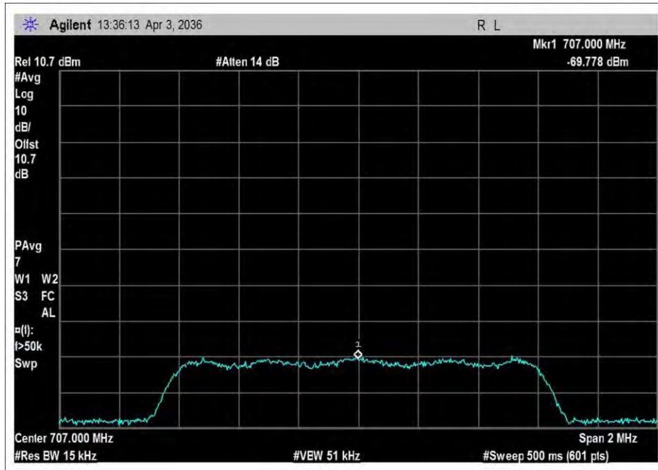
UL_698-716_input_CDMA
