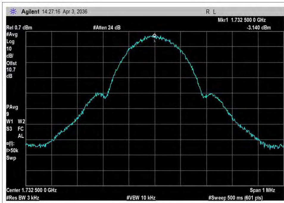
UL_1710-1755_output_GSM
