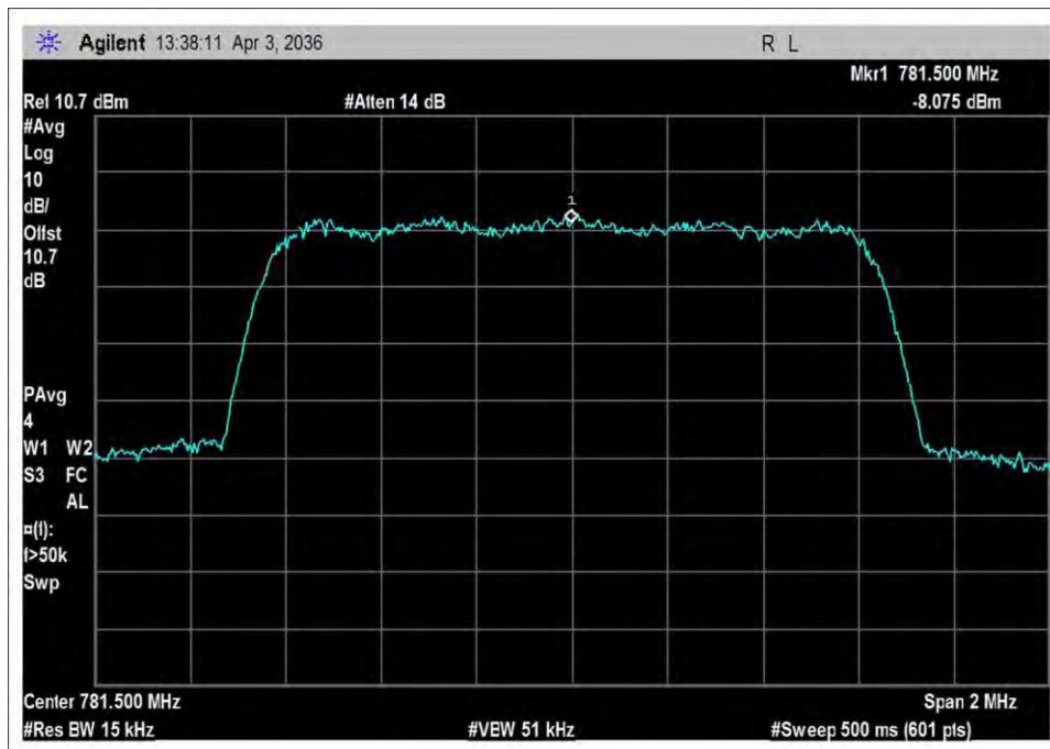
UL_776-787_output_CDMA
