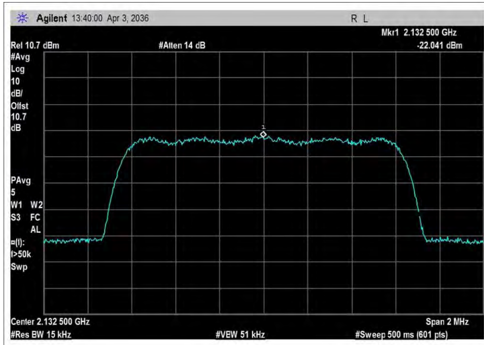
DL_2110-2155_output_CDMA
