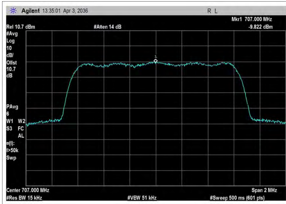
UL_698-716_output_CDMA
