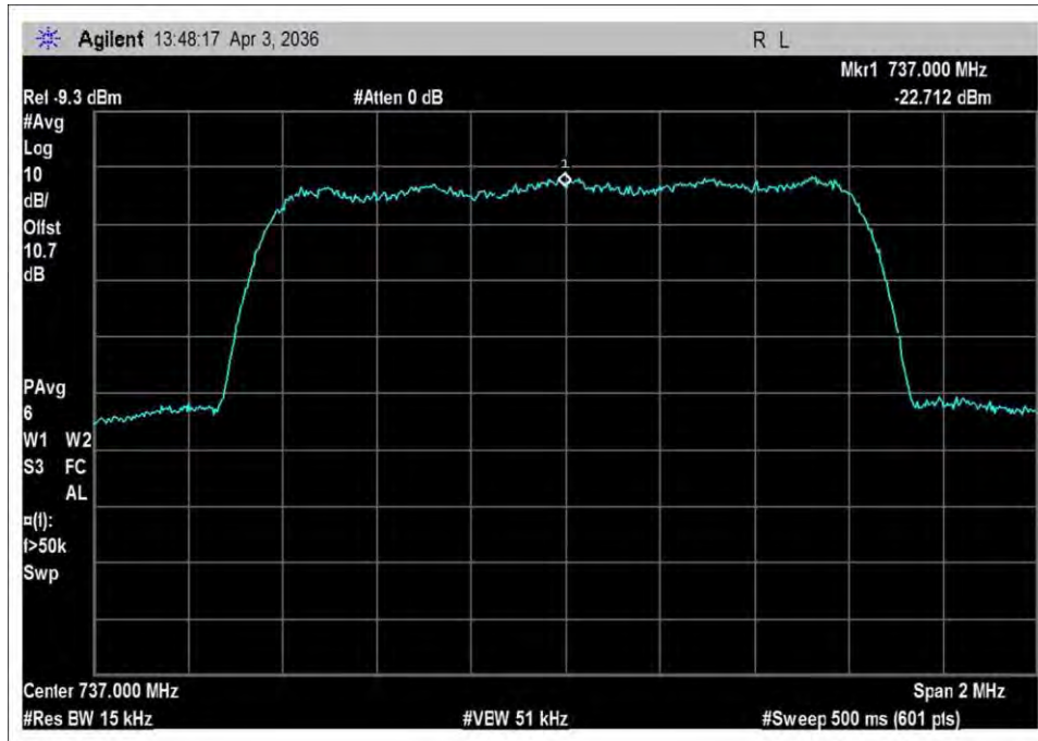
DL_728-746_output_CDMA
