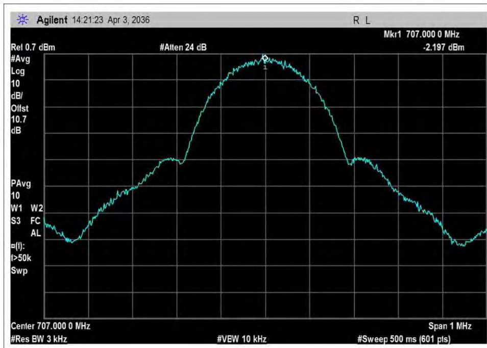
UL_698-716_output_GSM
