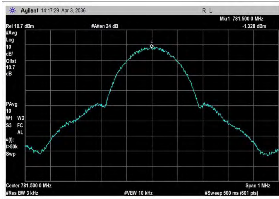
UL_776-787_output_GSM
