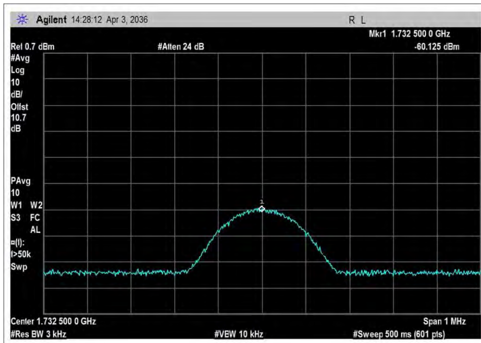
UL_1710-1755_input_GSM
