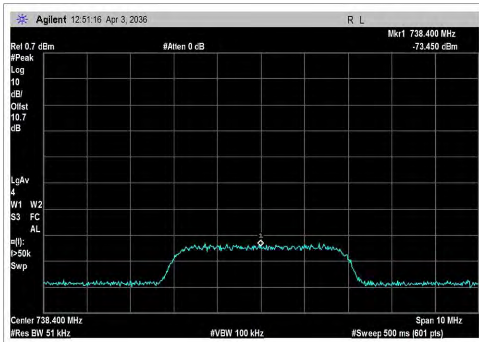
DL_728-746_input_WCDMA
