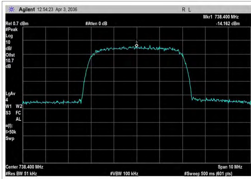
DL_728-746_output_WCDMA
