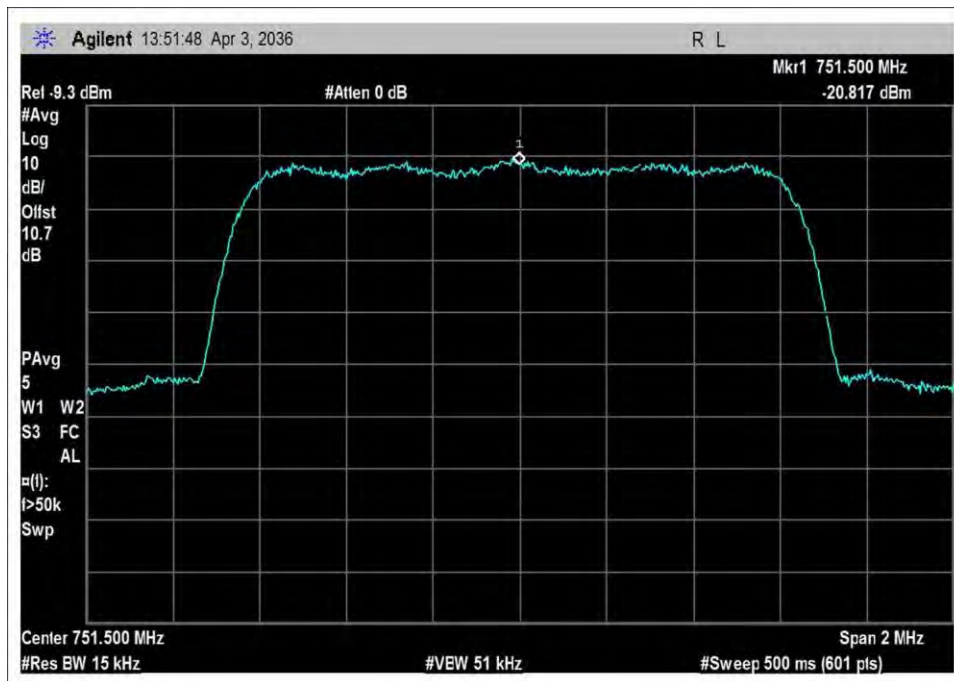
DL_746-757_output_CDMA
