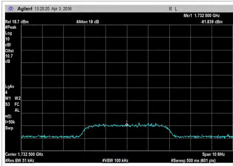
UL_1710-1755_input_WCDMA
