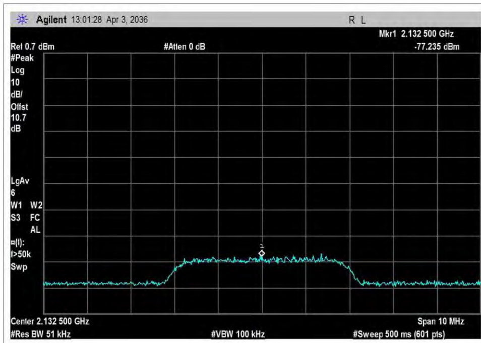
DL_2110-2155_input_WCDMA
