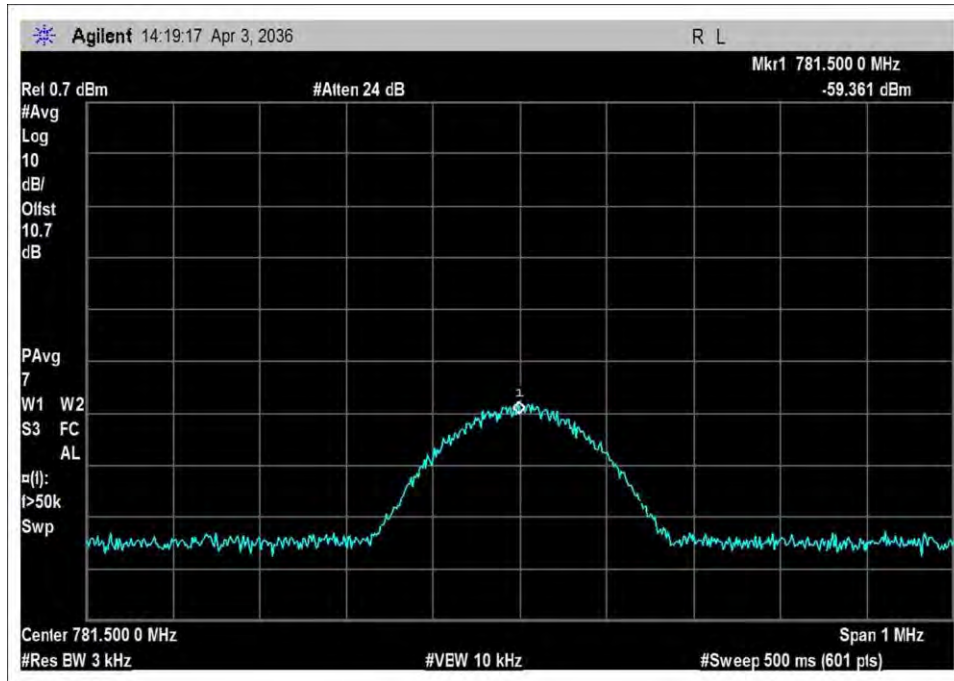
UL_776-787_input_GSM
