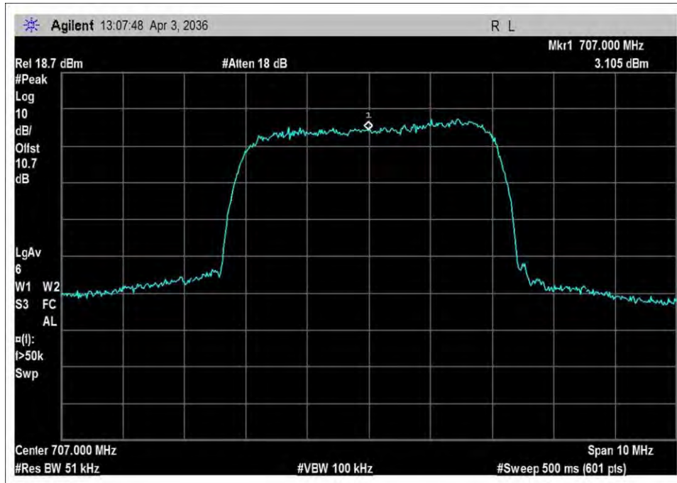
UL_698-716_output_WCDMA
