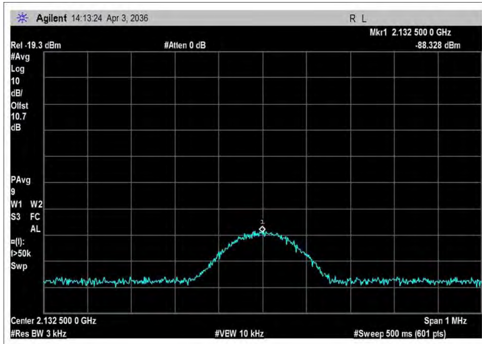
DL_2110-2155_input_GSM
