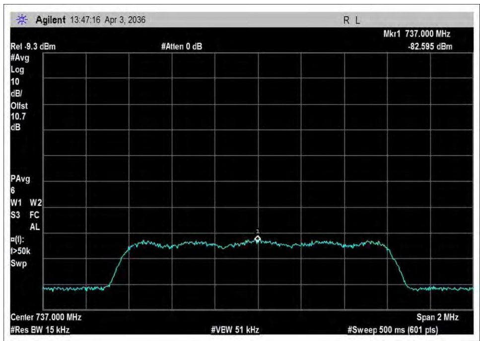
DL_728-746_input_CDMA
