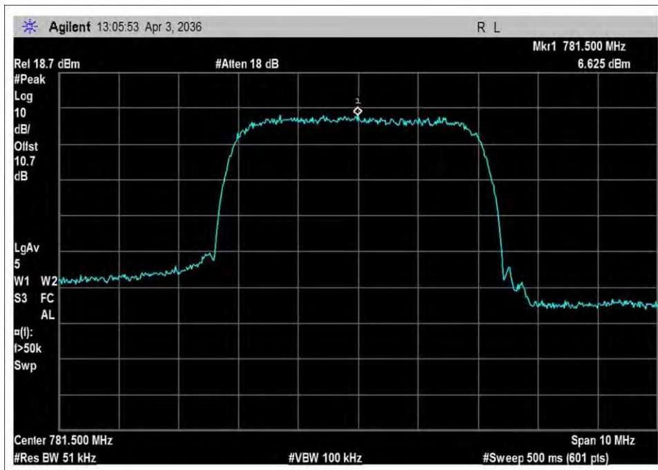
UL_776-787_output_WCDMA
