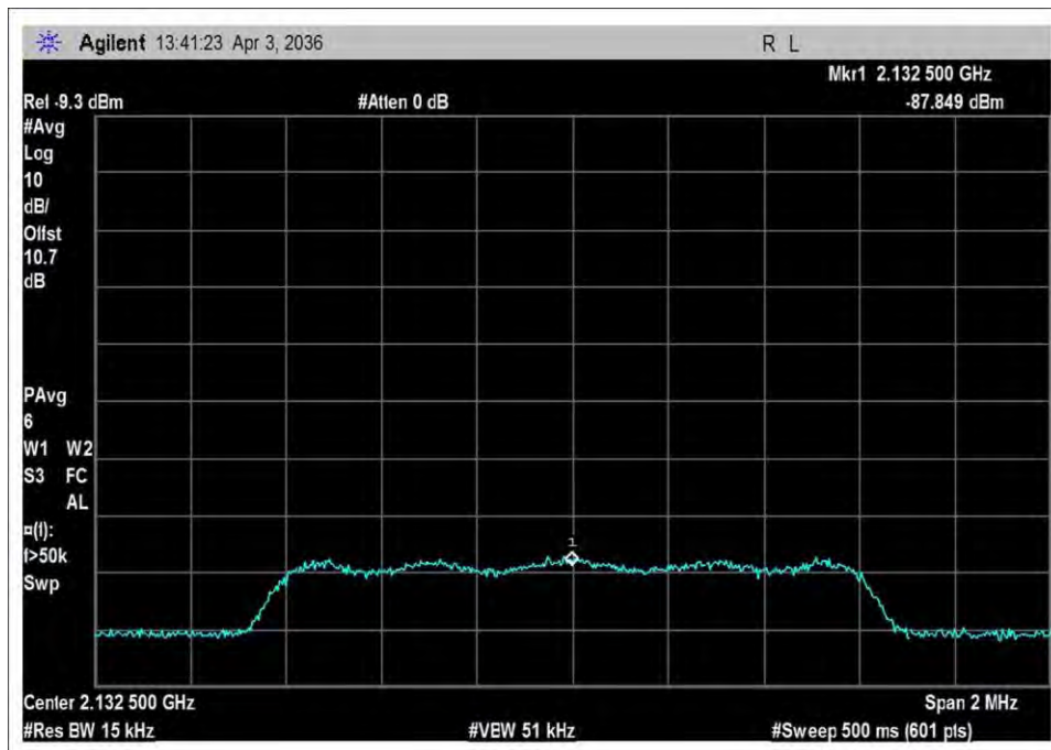
DL_2110-2155_input_CDMA
