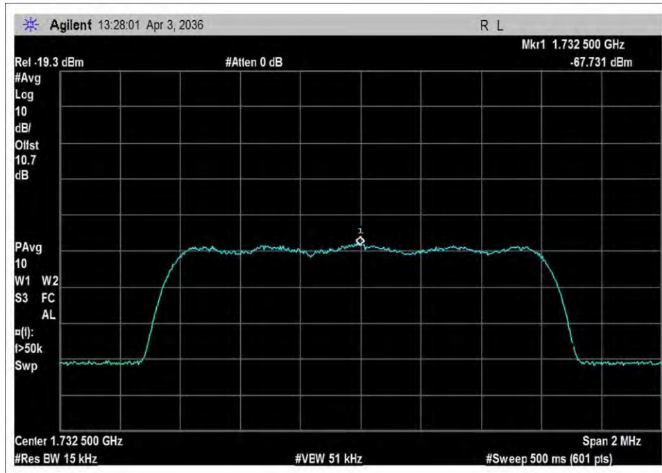
UL_1710-1755_input_CDMA
