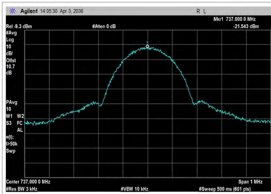
DL_728-746_output_GSM
