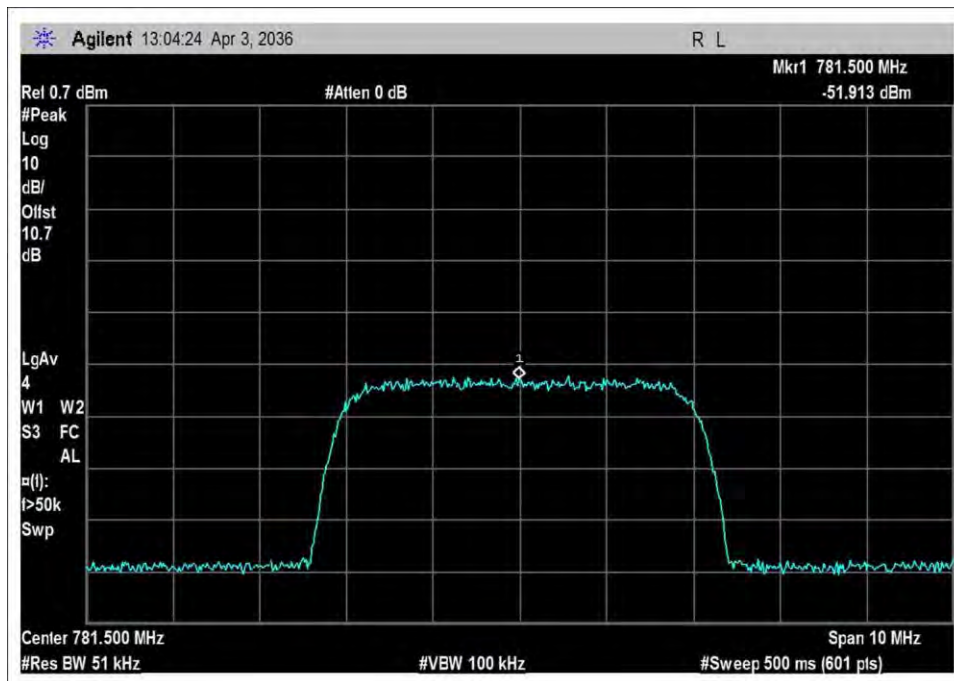
UL_776-787_input_WCDMA
