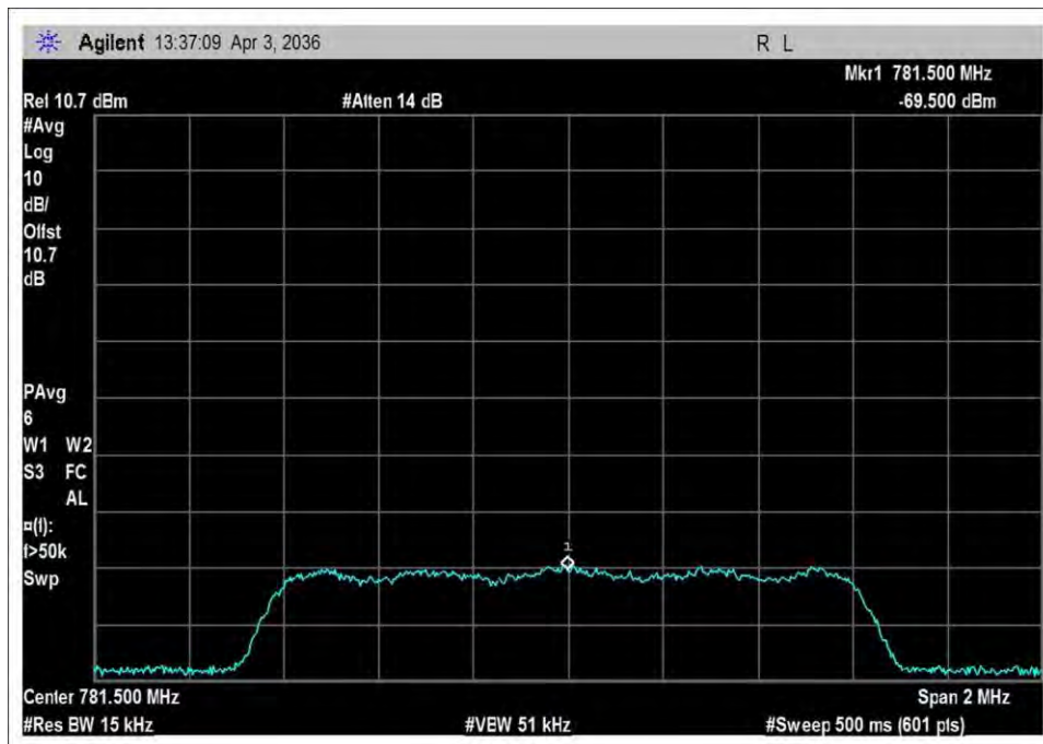
UL_776-787_input_CDMA
