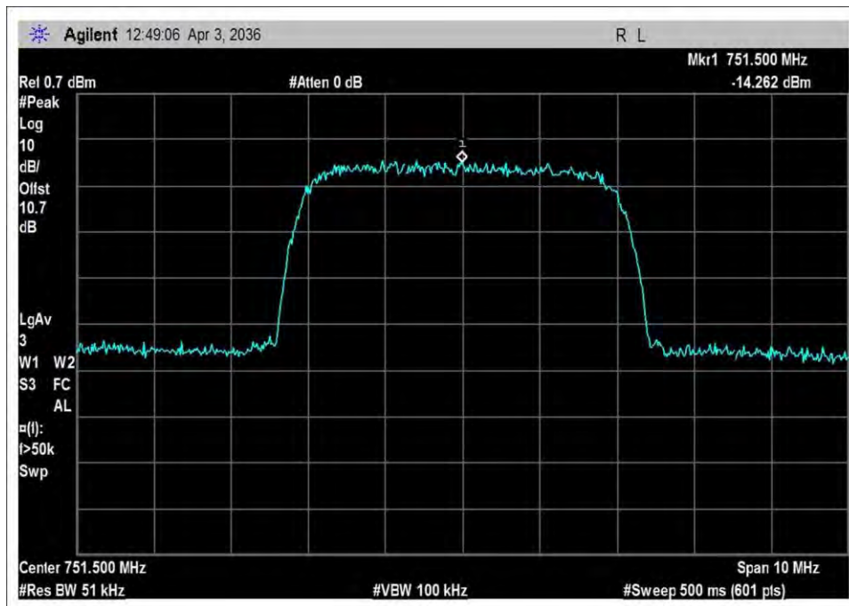
DL_746-757_output_WCDMA
