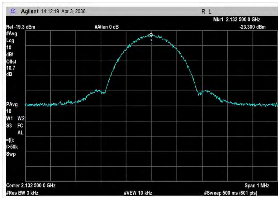
DL_2110-2155_output_GSM
