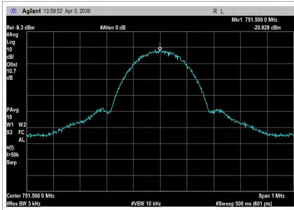
DL_746-757_output_GSM
