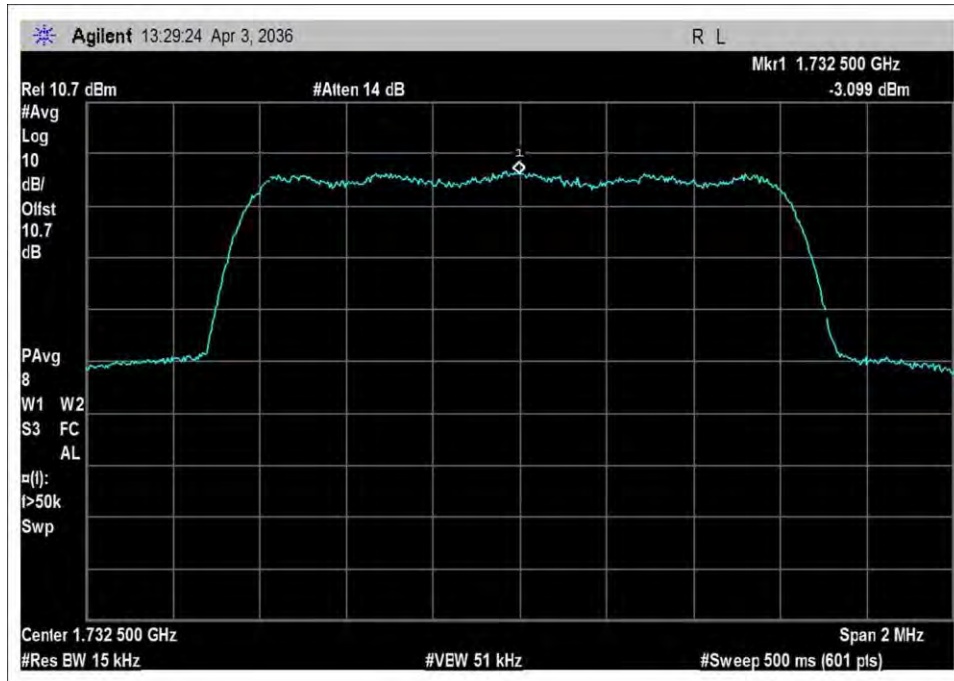
UL_1710-1755_output_CDMA
