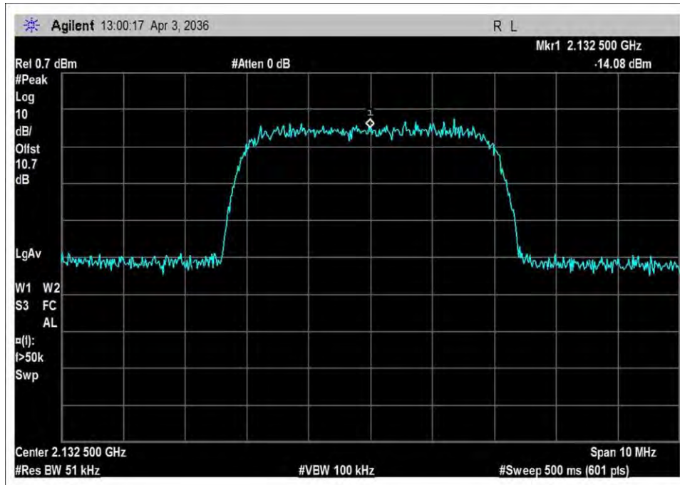
DL_2110-2155_output_WCDMA
