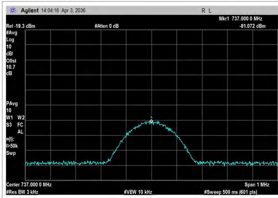
DL_728-746_input_GSM
