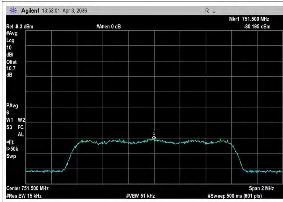
DL_746-757_input_CDMA
