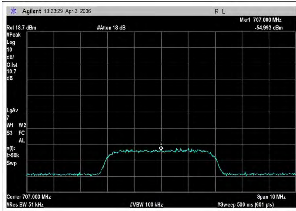
UL_698-716_input_WCDMA
