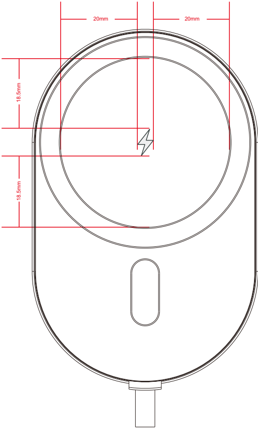
闪电符号镭雕位置
