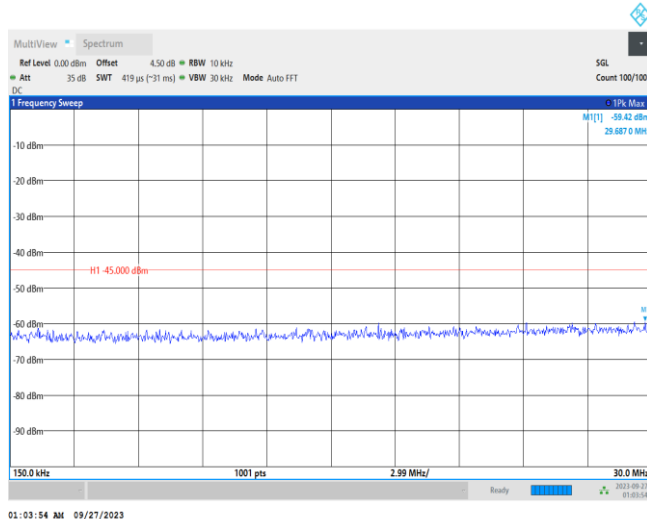
Band38-20MHz-QPSK-37850-1RB#0-Range2:0.15~30MHz
