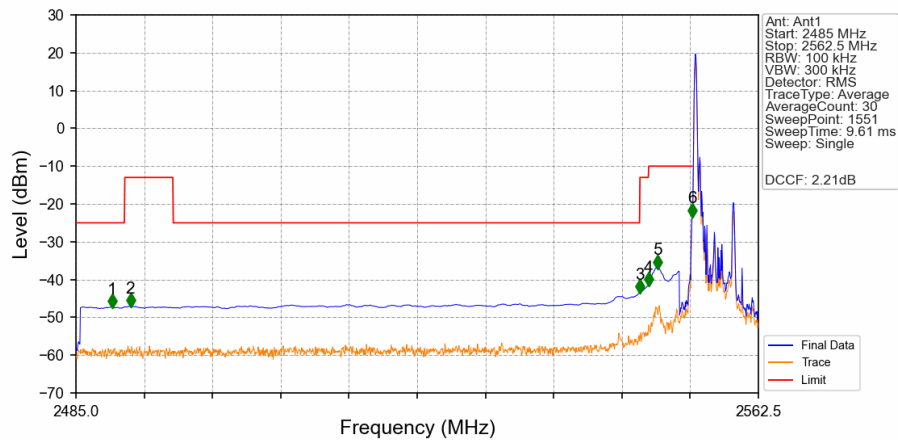
Band41_5MHz_QPSK_LCH_2557.5MHz_RB_1_0_NTNV
