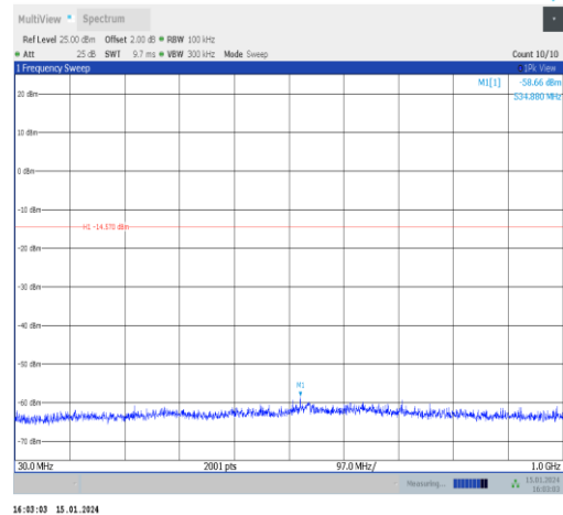
11g-Ant1-2437-30~1000-PASS
