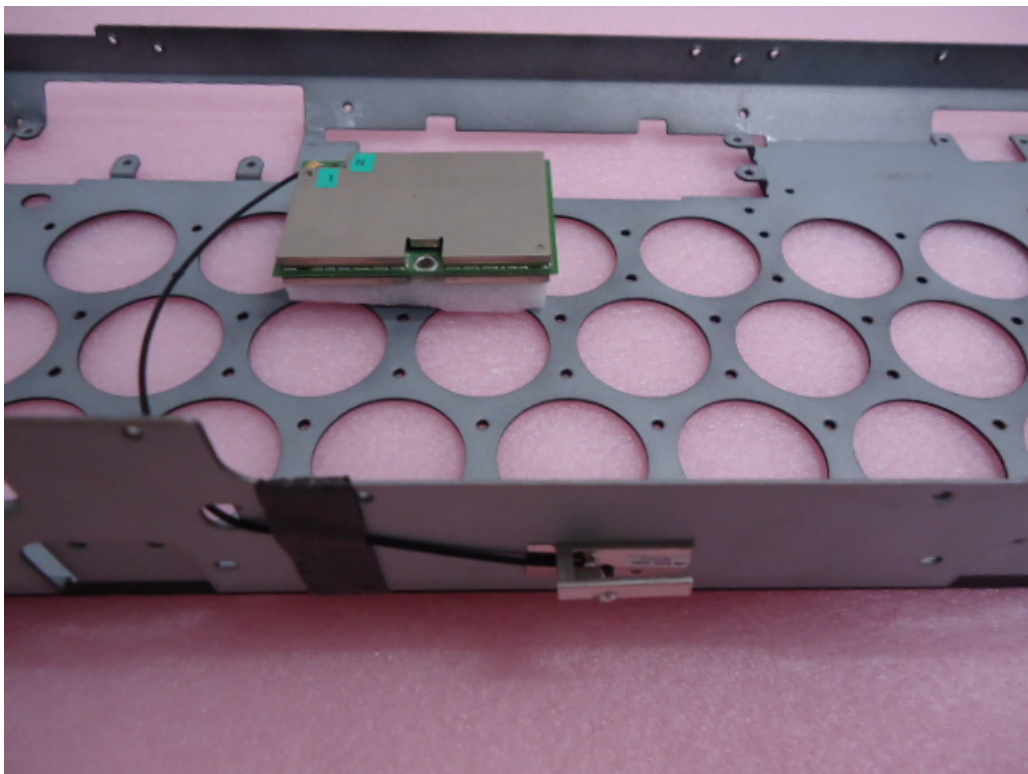
81EAAY15.G09(PIFA) Closeup
