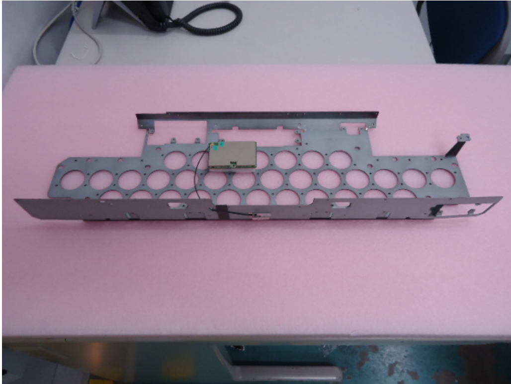
81EAAY15.G09(PIFA) Whole
