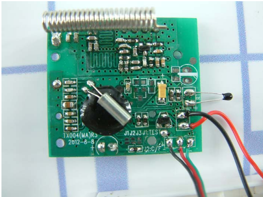
TX PCB1 side1
