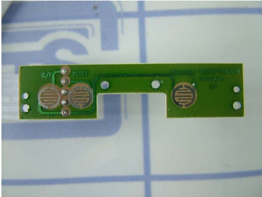
PCB2 side2
