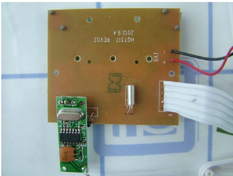
PCB1 side1
