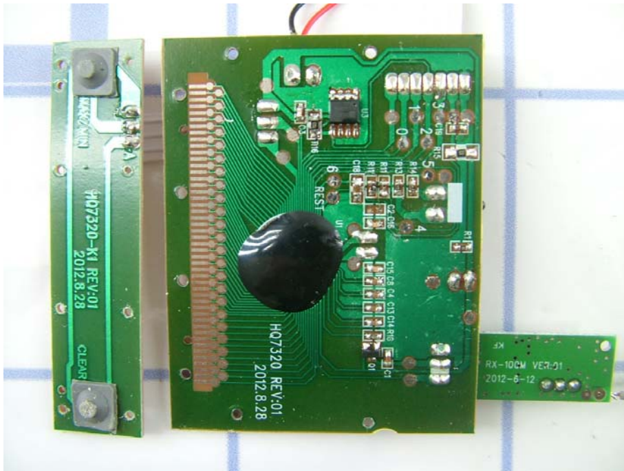
PCB1 side2
