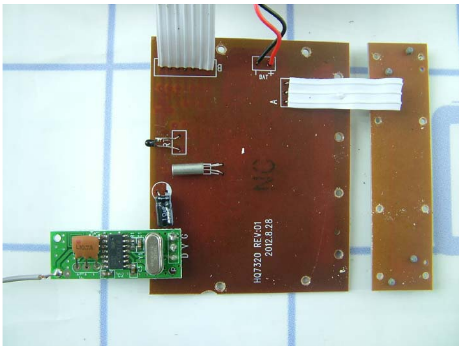
PCB1 side1
