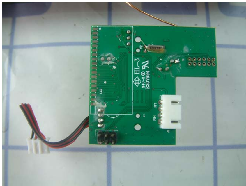
PCB2 side2
