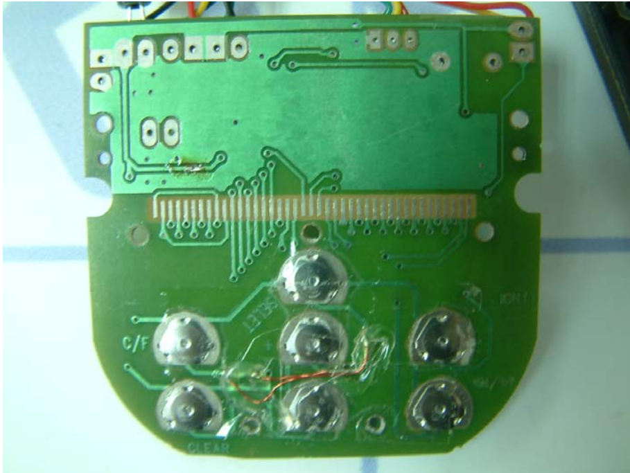
RX PCB2 side2
