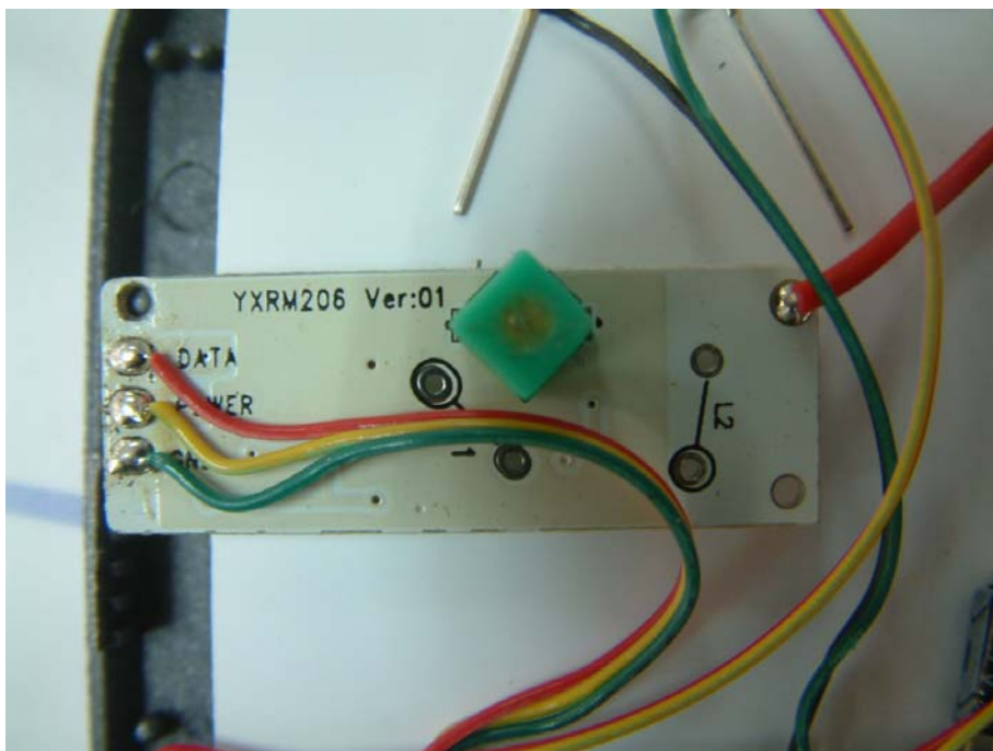
RX PCB1 side1
