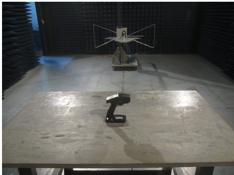
SE 30MHz-1GHz
