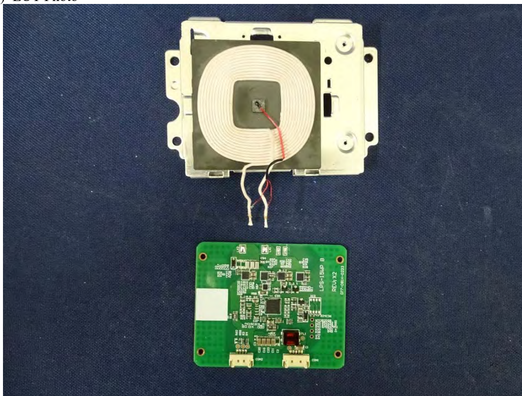
(48) EUT Photo
