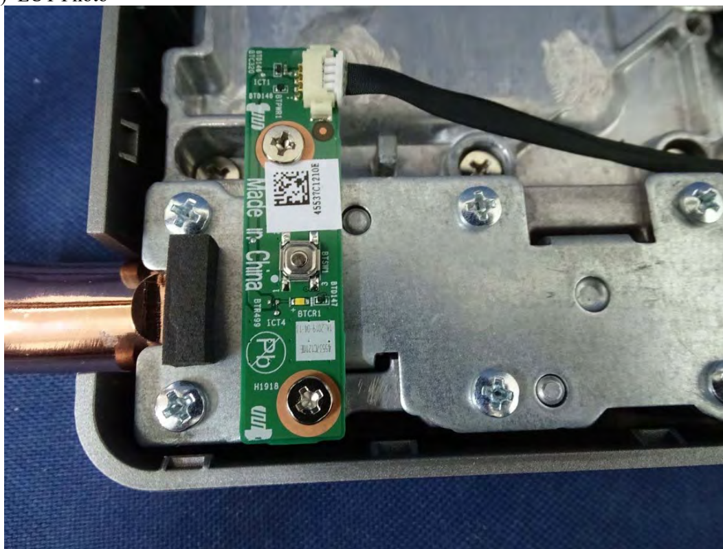
(40) EUT Photo
