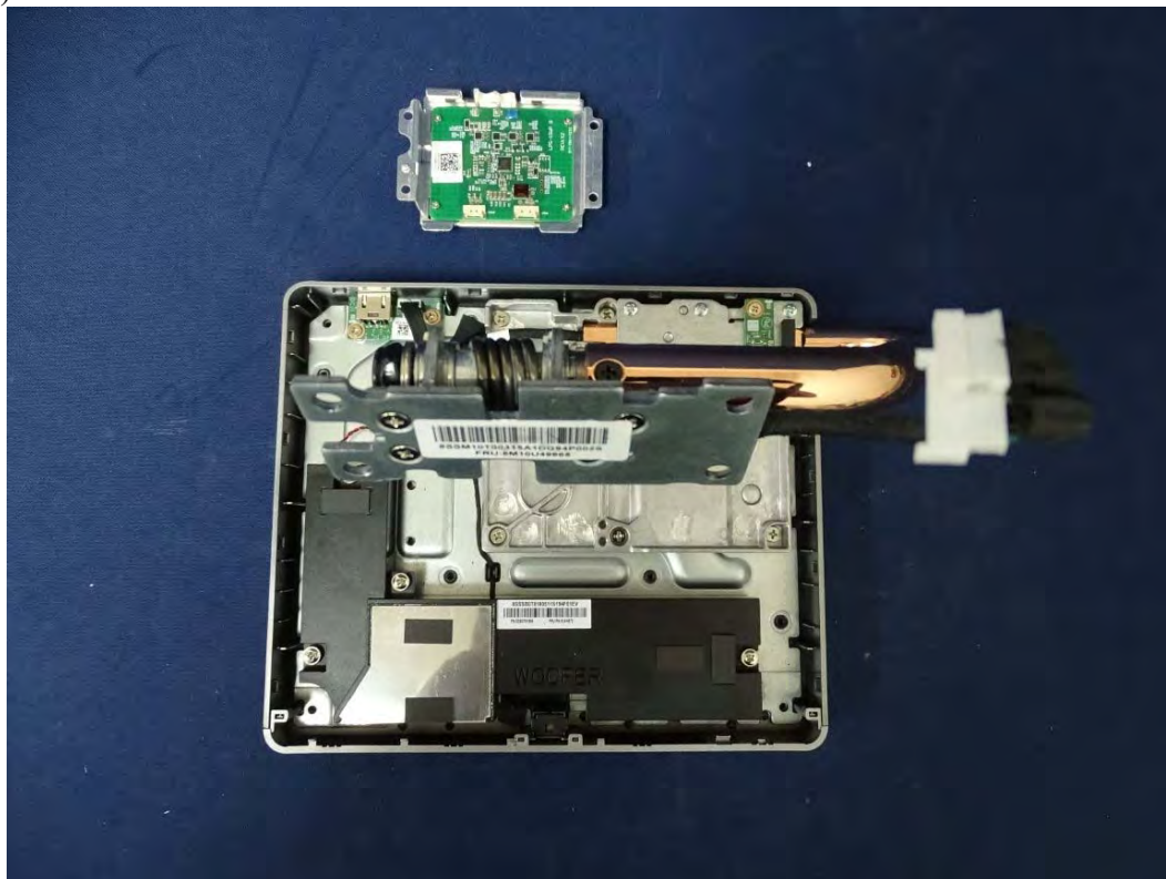
(40) EUT Photo
