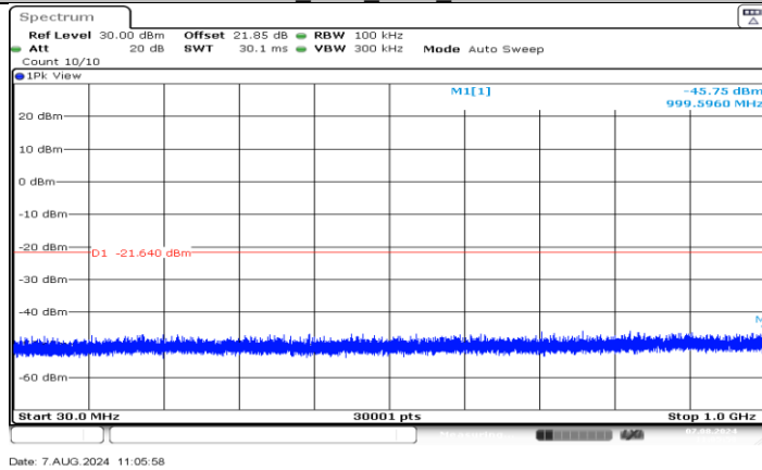
SRD 2.4G_Ant1_2480_30-1000
