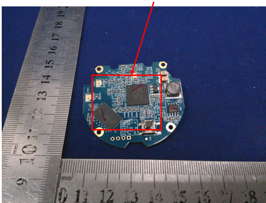
Wifi Module
