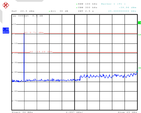
30MHz~25GHz
