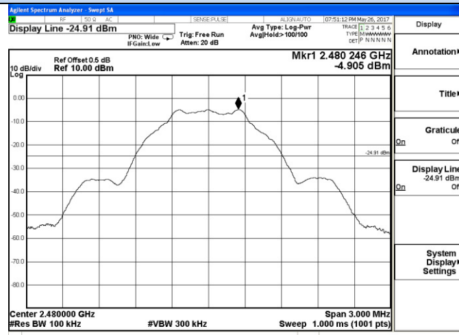
2479 – 2481 MHz
