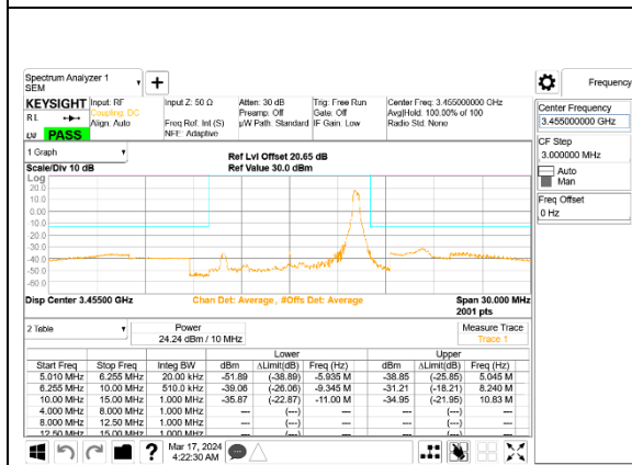
5G NR n77 10MHz BPSK Low Channel RB1-23, ID:28498
