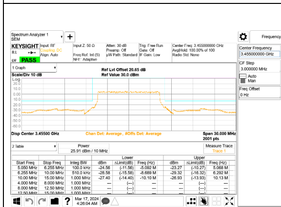
5G NR n77 10MHz BPSK Low Channel RB24-0, ID:28498
