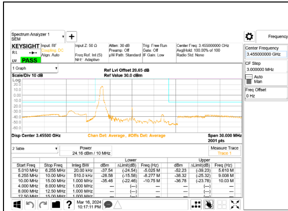
5G NR n77 10MHz BPSK Low Channel RB1-0, ID:28498
