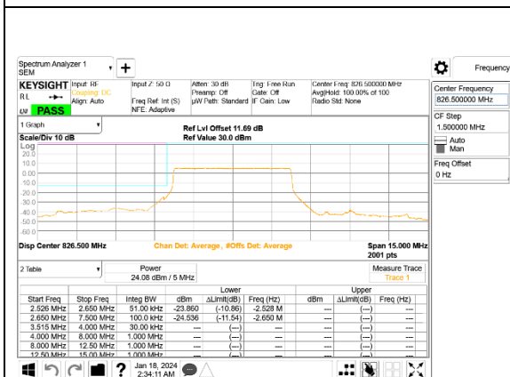
5G NR n5 5MHz BPSK Low Channel RB25-0, ID:24898
