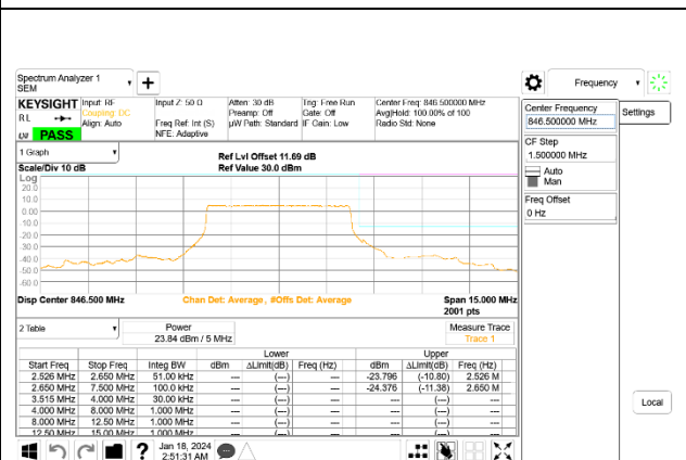
5G NR n5 5MHz BPSK High Channel RB25-0, ID:24898
