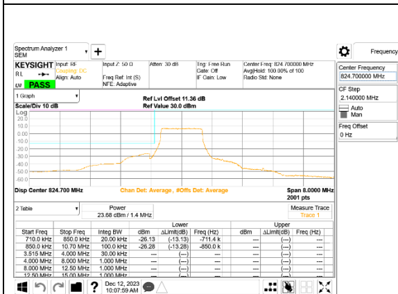
LTE B5 1.4MHz QPSK Low Channel RB6-0, ID:32061
