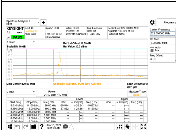
5G NR n5 10MHz BPSK Low Channel RB1-0, ID:24898
