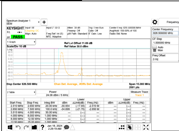
5G NR n5 5MHz BPSK Low Channel RB1-0, ID:24898
