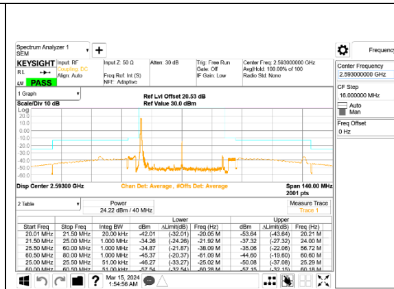
5G NR n41 40MHz BPSK Middle Channel RB1-0, ID:24898
