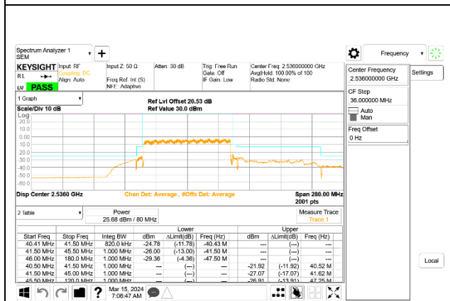
5G NR n41 80MHz BPSK Low Channel RB216-0, ID:24898
