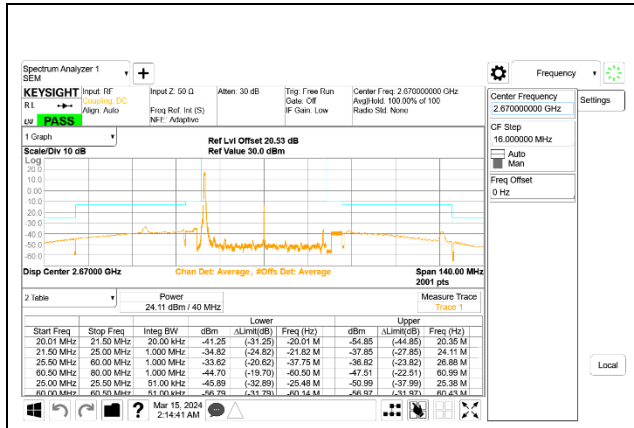
5G NR n41 40MHz BPSK High Channel RB1-0, ID:24898
