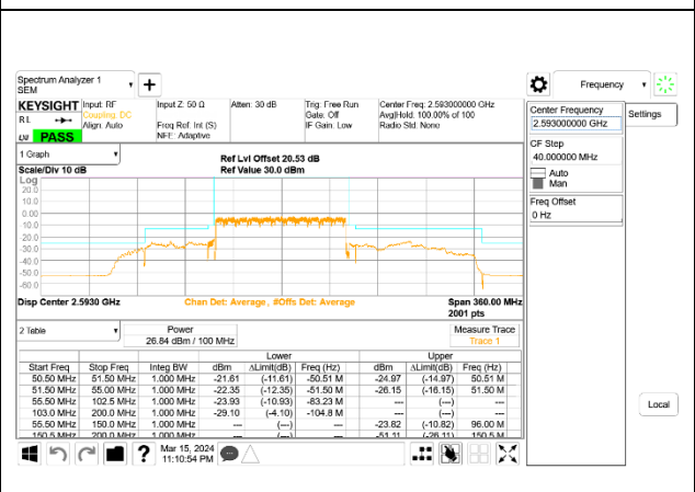
5G NR n41 100MHz BPSK Middle Channel RB270-0, ID:24898
