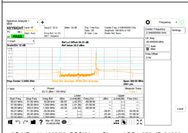
5G NR n41 100MHz BPSK Low Channel RB1-272, ID:24898
