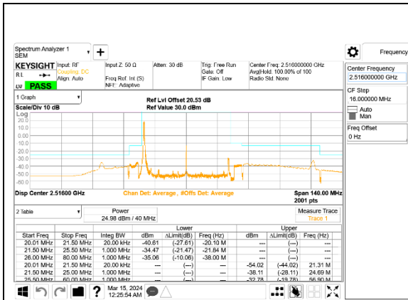
5G NR n41 40MHz BPSK Low Channel RB1-0, ID:24898
