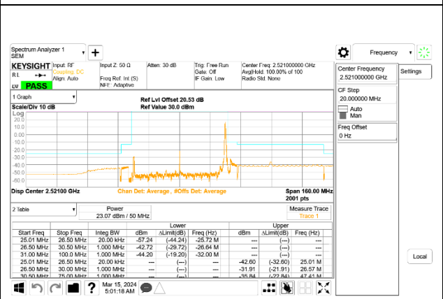
5G NR n41 50MHz BPSK Low Channel RB1-132, ID:24898
