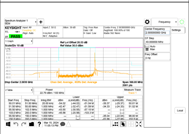
5G NR n41 100MHz BPSK Middle Channel RB1-272, ID:24898
