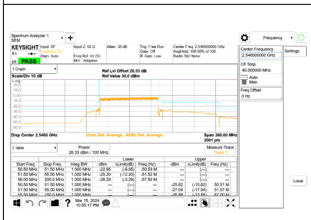
5G NR n41 100MHz BPSK Low Channel RB270-0, ID:24898
