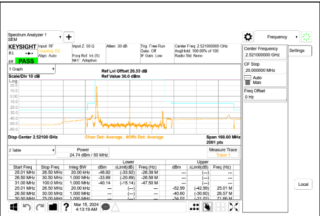
5G NR n41 50MHz BPSK Low Channel RB1-0, ID:24898
