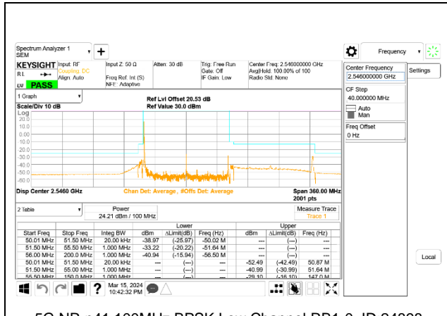
5G NR n41 100MHz BPSK Low Channel RB1-0, ID:24898
