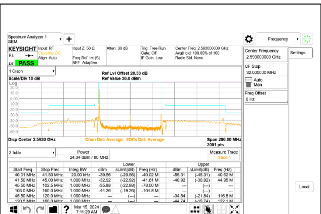
5G NR n41 80MHz BPSK Middle Channel RB1-0, ID:24898
