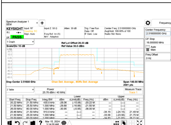
5G NR n41 40MHz BPSK Low Channel RB100-0, ID:24898
