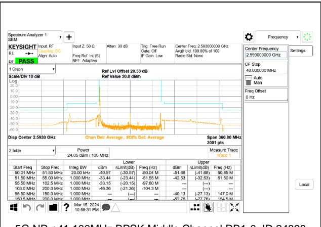
5G NR n41 100MHz BPSK Middle Channel RB1-0, ID:24898
