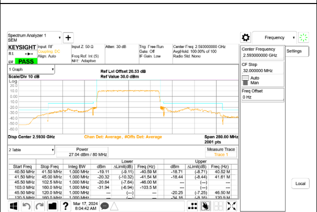
5G NR n41 80MHz BPSK Middle Channel RB216-0, ID:24898
