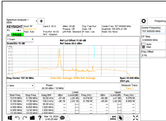
5G NR n12 10MHz BPSK Middle Channel RB1-0, ID:28498
