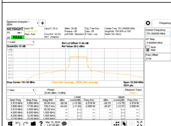
5G NR n12 5MHz BPSK Low Channel RB25-0, ID:28498
