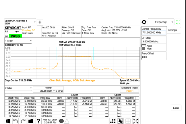
5G NR n12 10MHz BPSK High Channel RB50-0, ID:28498
