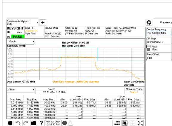
5G NR n12 10MHz BPSK Middle Channel RB50-0, ID:28498
