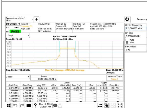
5G NR n12 5MHz BPSK High Channel RB25-0, ID:28498
