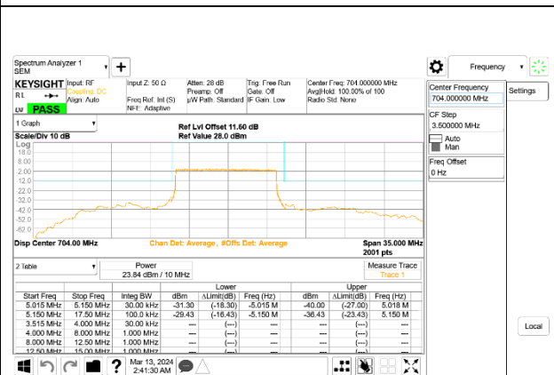
5G NR n12 10MHz BPSK Low Channel RB50-0, ID:28498
