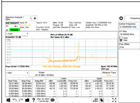
5G NR n77 50MHz BPSK Low Channel RB1-132, ID:28498
