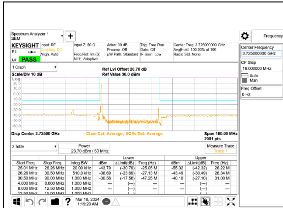
5G NR n77 50MHz BPSK Low Channel RB1-0, ID:28498
