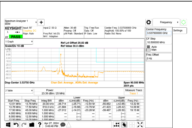
5G NR n77 25MHz BPSK High Channel RB1-0, ID:28498
