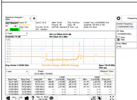
5G NR n77 50MHz BPSK High Channel RB1-132, ID:28498
