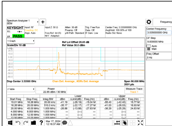
5G NR n77 30MHz BPSK High Channel RB1-0, ID:28498
