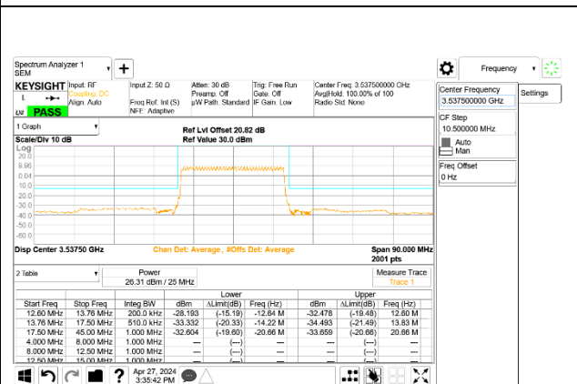
5G NR n77 25MHz BPSK High Channel RB64-0, ID:28498
