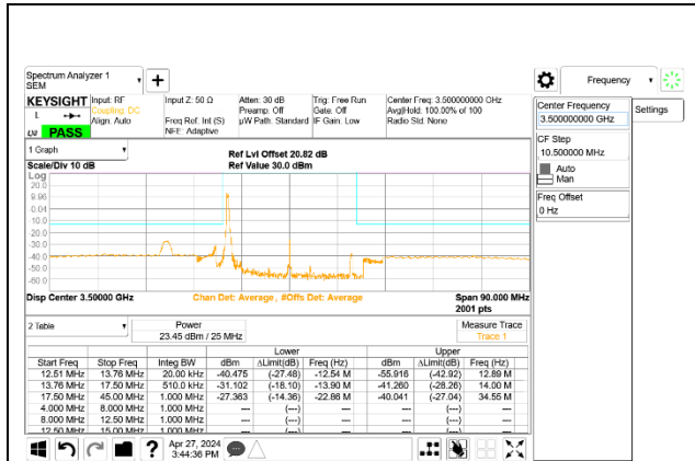
5G NR n77 25MHz BPSK Middle Channel RB1-0, ID:28498
