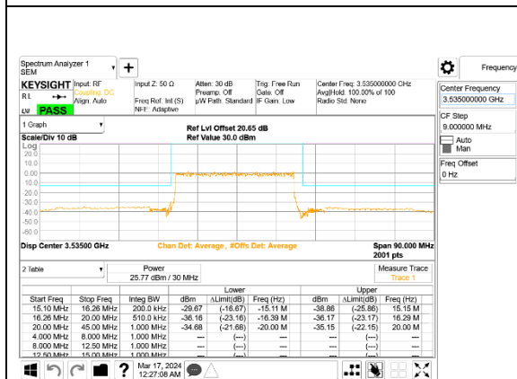
5G NR n77 30MHz BPSK High Channel RB75-0, ID:28498
