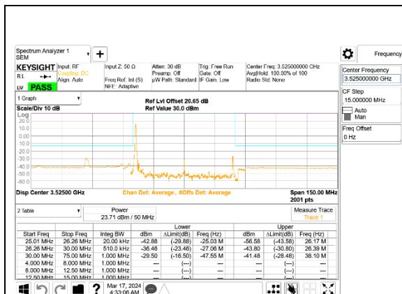
5G NR n77 50MHz BPSK High Channel RB1-0, ID:28498
