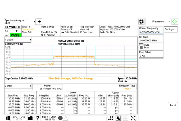
5G NR n77 60MHz BPSK Low Channel RB162-0, ID:28498
