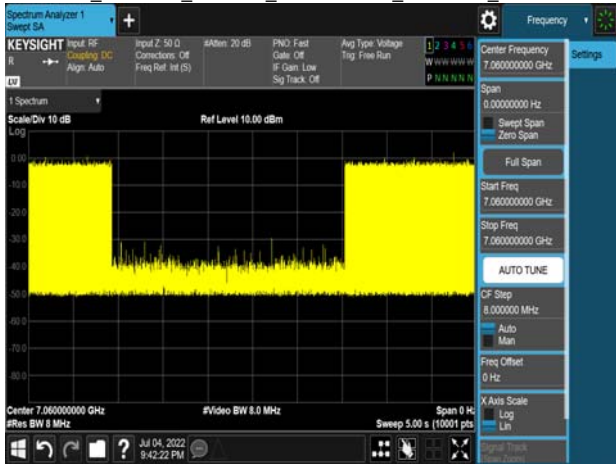
Det Lel_802.11ax_160MHz_CF 6985MHz_7060MHz_-71.18dBm
