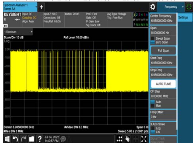
Det Lel_802.11ax_160MHz_CF 6985MHz_6985MHz_-68.35dBm
