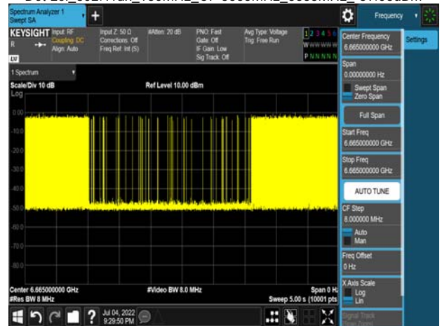
Det Le1_802.11ax_160MHz_CF 6665MHz_6665MHz_-69.06dBm
