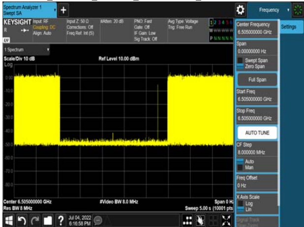
Det Lel_802.11ax_160MHz_CF 6505MHz_6430MHz-73.17dBm
