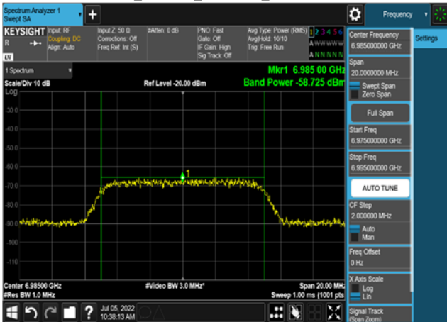
802.11ax_160MHz_6985MHz_AWGN:6985MHz
