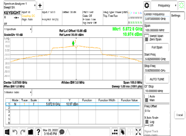
802.11n_40MHz_Chain1_5875MHz
