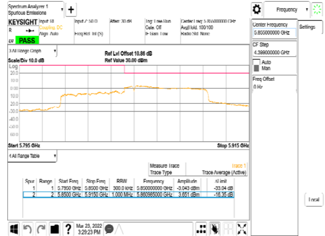
802.11ac_80MHz_Chain1_5855MHz
