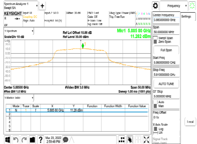
802.11n_20MHz_Chain1_5885MHz
