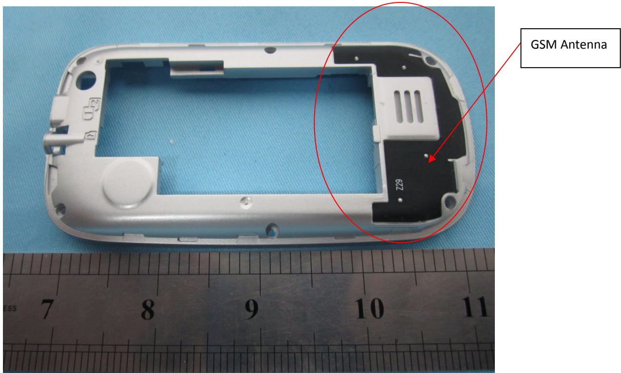
GSM Antenna
