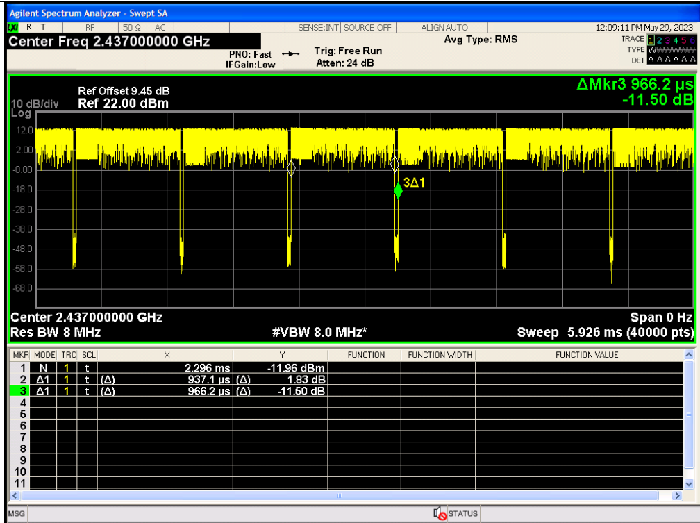
IEEE 802.11b_20MHz_Channel 6
