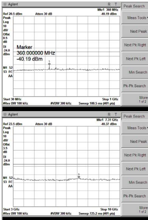
802.11 n(20M) Mode, Ch6
