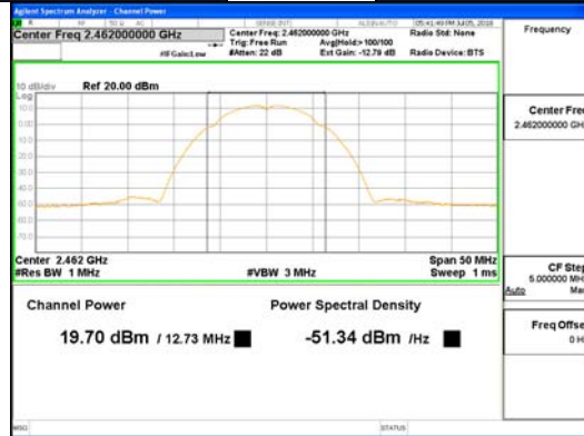
802.11b_ANT3
