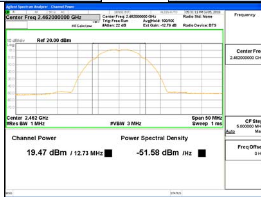
802.11b_ANT2
