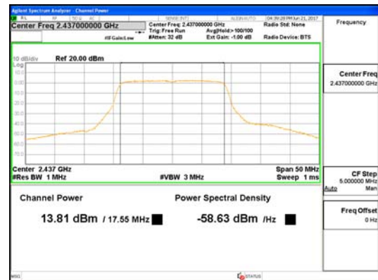
Ant 0_802.11n_HT20
