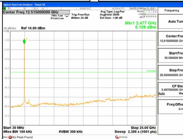
Ant 2_802.11n_HT20
