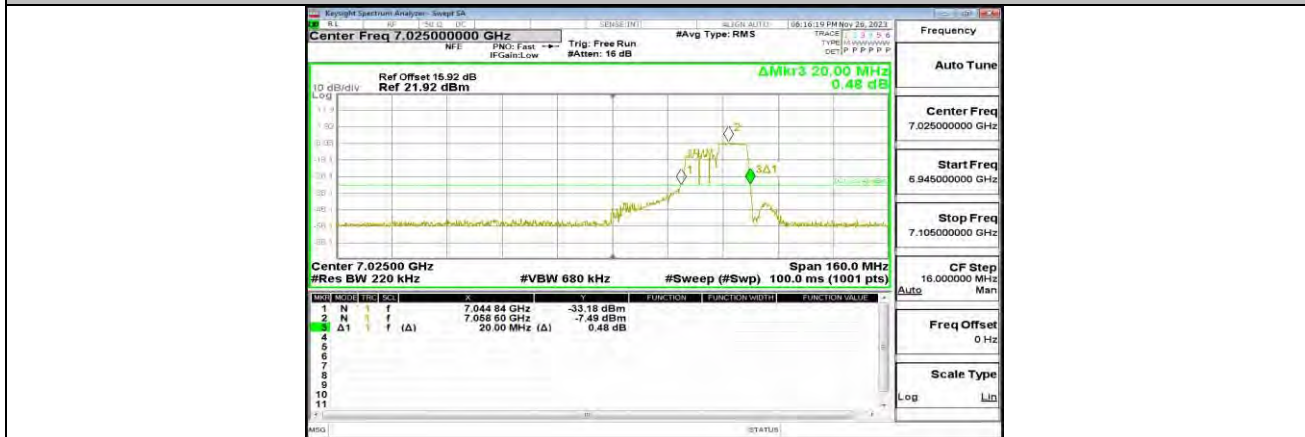
11AX80MIMO_ANT0_7025_106Tone_RU60
