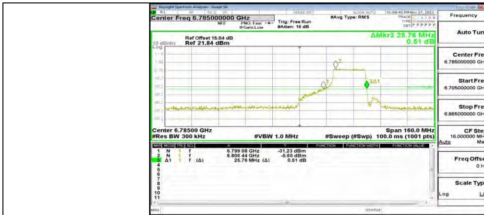
11AX80MIMO_ANT1_6785_242Tone_RU64
