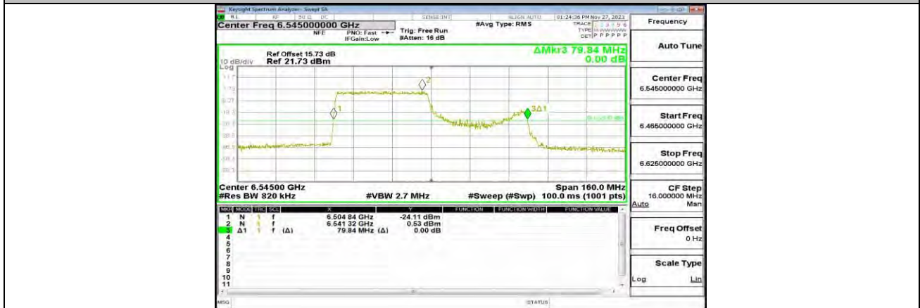
11AX80MIMO_ANT0_6545_242Tone_RU64
