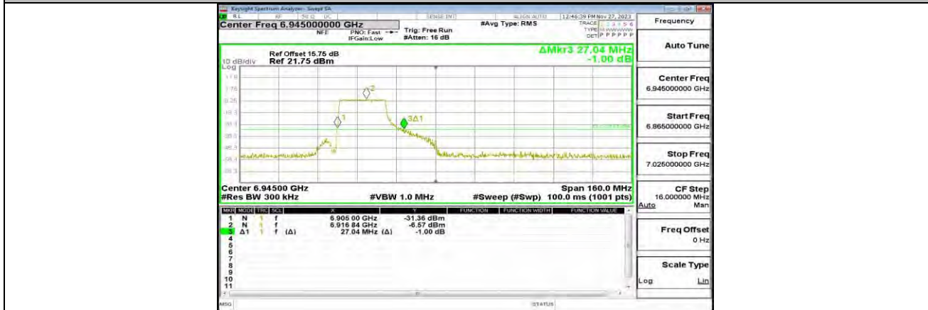
11AX80MIMO_ANT0_6945_242Tone_RU61
