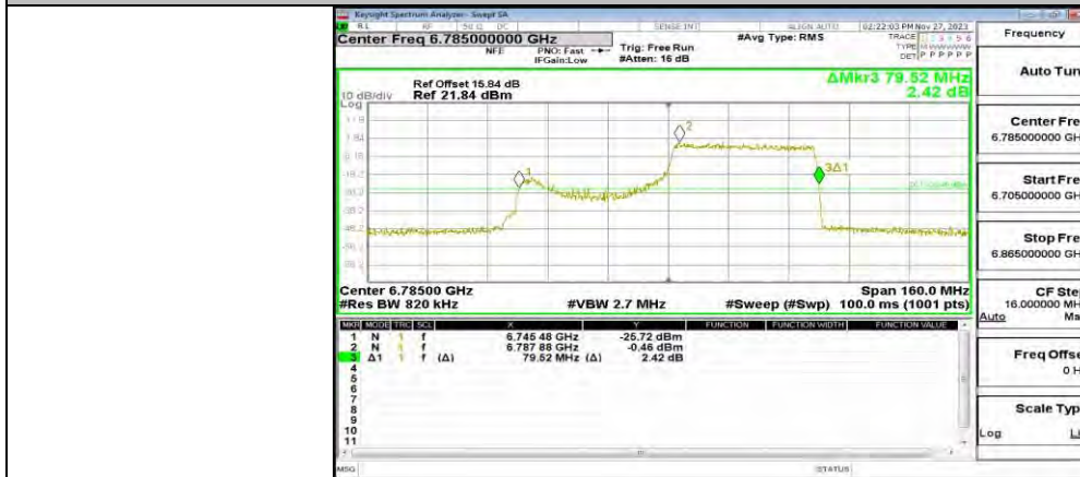
11AX80MIMO_ANT1_6785_484Tone_RU66
