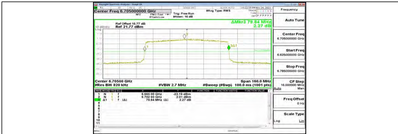
11AX80MIMO_ANT0_6705_996Tone_RU67
