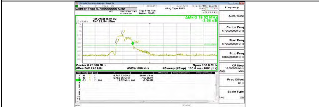
11AX80MIMO_ANT1_6785_106Tone_RU53
