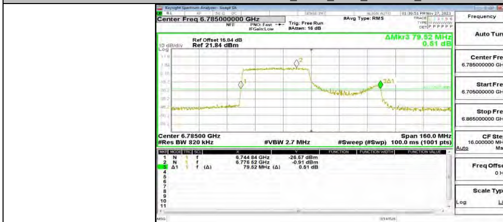
11AX80MIMO_ANT1_6785_484Tone_RU65
