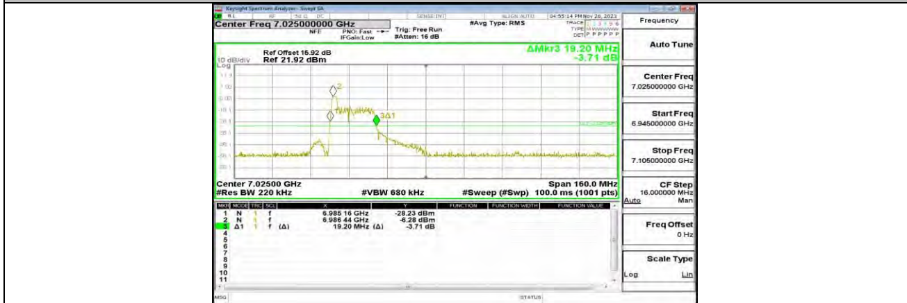
11AX80MIMO_ANT0_7025_26Tone_RU0
