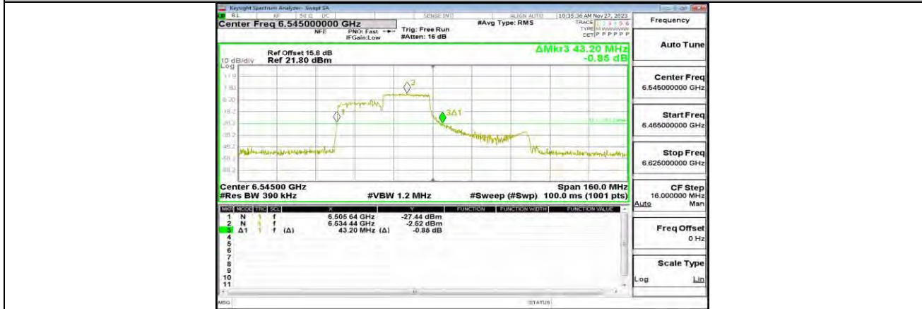
11AX80MIMO_ANT1_6545_242Tone_RU62
