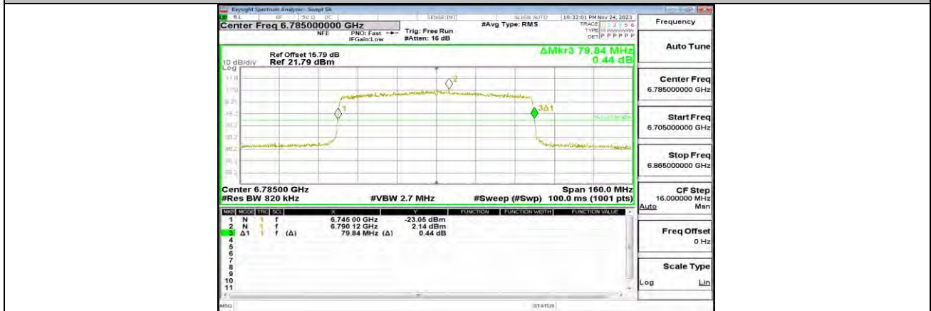
11AX80MIMO_ANT0_6785_996Tone_RU67
