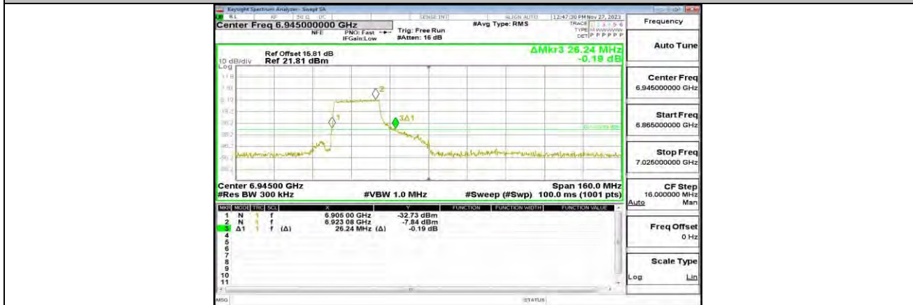
11AX80MIMO_ANT1_6945_242Tone_RU61
