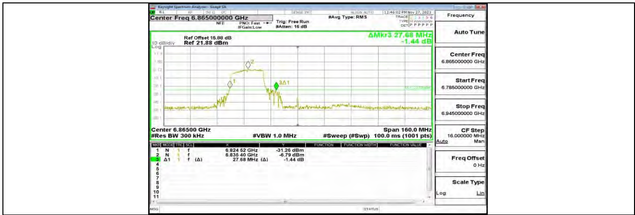
11AX80MIMO_ANT1_6865_242Tone_RU61
