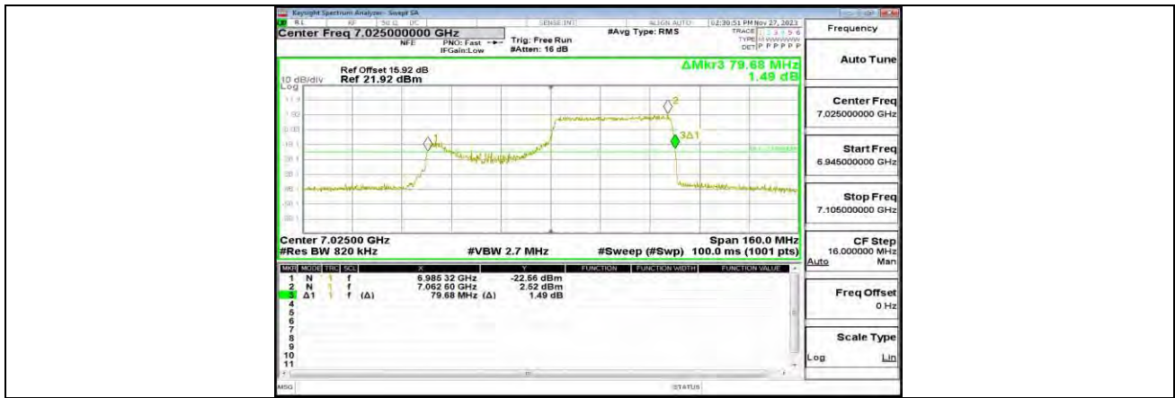
11AX80MIMO_ANT0_7025_484Tone_RU66
