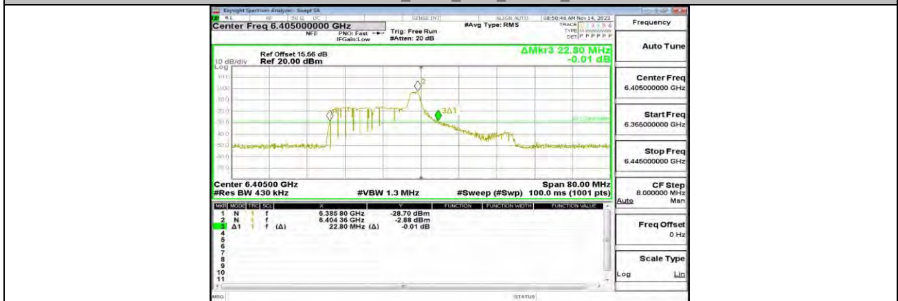
11AX40MIMO_ANT0_6405_26Tone_RU0
