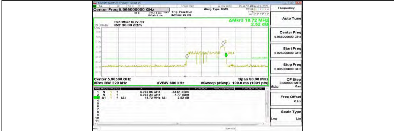
11AX40MIMO_ANT1_5965_26Tone_RU8
