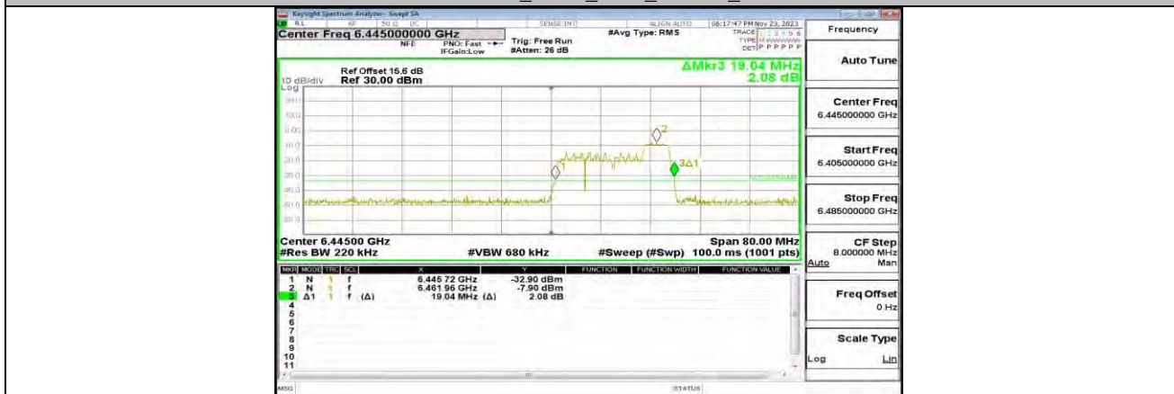
11AX40MIMO_ANT0_6445_52Tone_RU40
