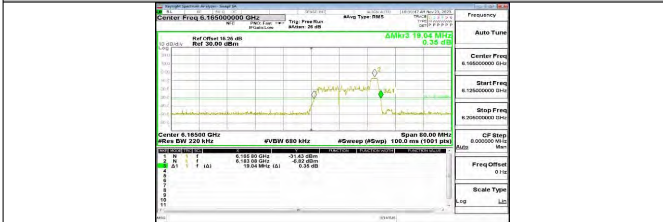
11AX40MIMO_ANT0_6165_26Tone_RU17
