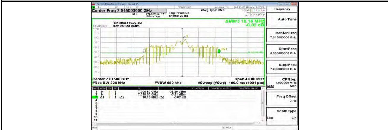
11AX20MIMO_ANT0_7015_26Tone_RU0
