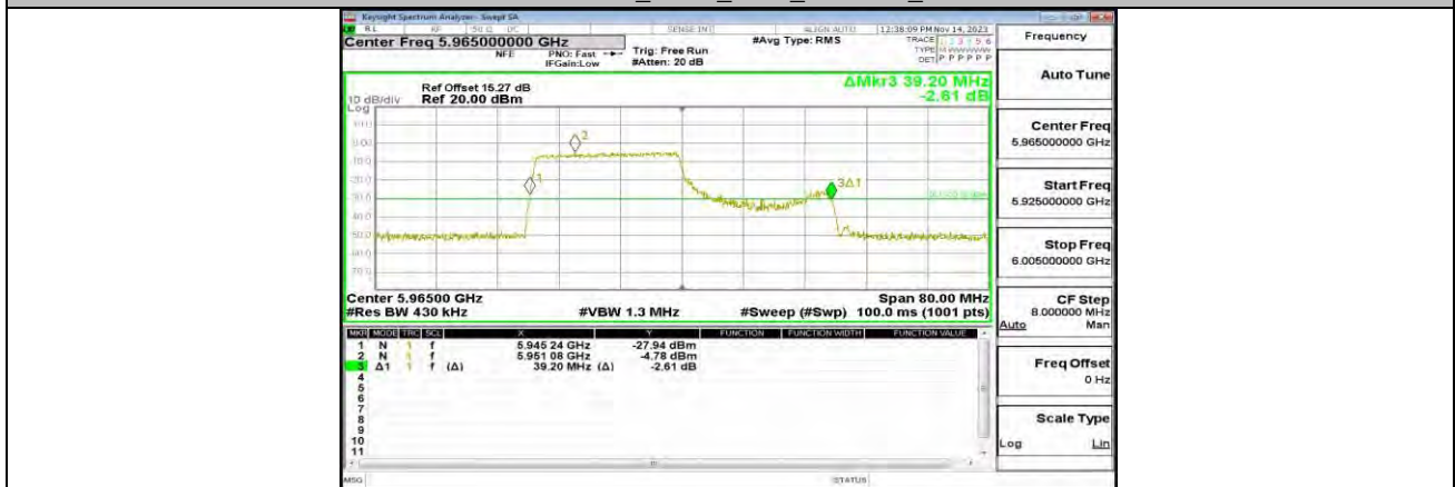
11AX40MIMO_ANT1_5965_106Tone_RU56
