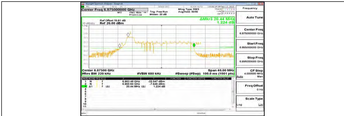
11AX20MIMO_ANT1_6875_26Tone_RU0
