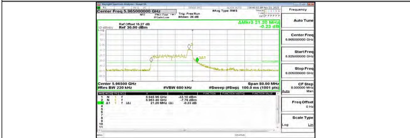
11AX40MIMO_ANT1_5965_26Tone_RU8
