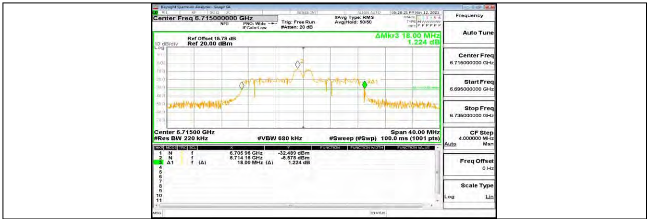
11AX20MIMO_ANT1_6715_26Tone_RU4
