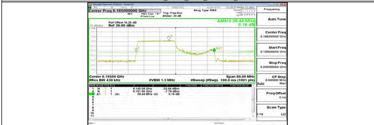
11AX40MIMO_ANT0_6165_242Tone_RU61
