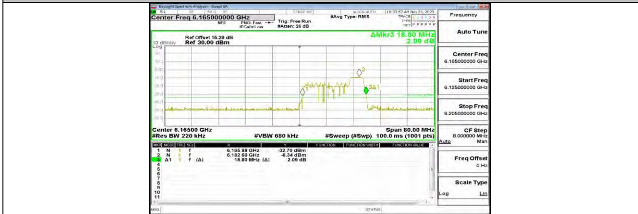
11AX40MIMO_ANT1_6165_52Tone_RU44
