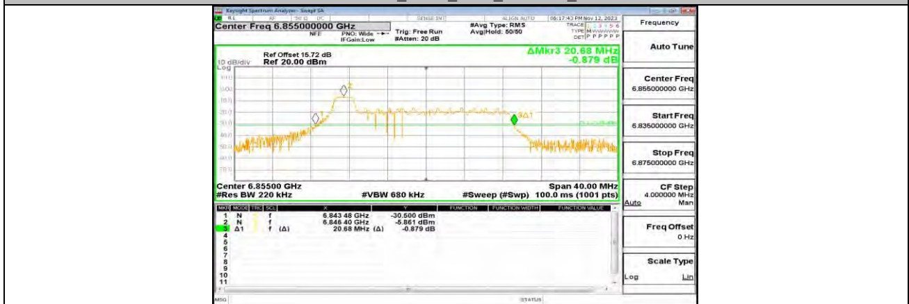
11AX20MIMO_ANT0_6855_26Tone_RU0
