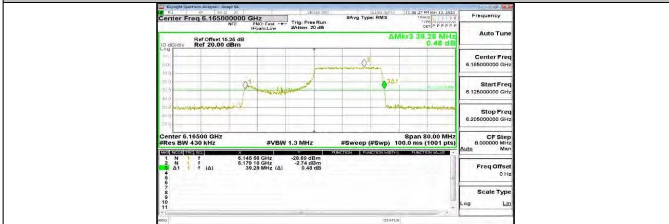
11AX40MIMO_ANT0_6165_242Tone_RU62
