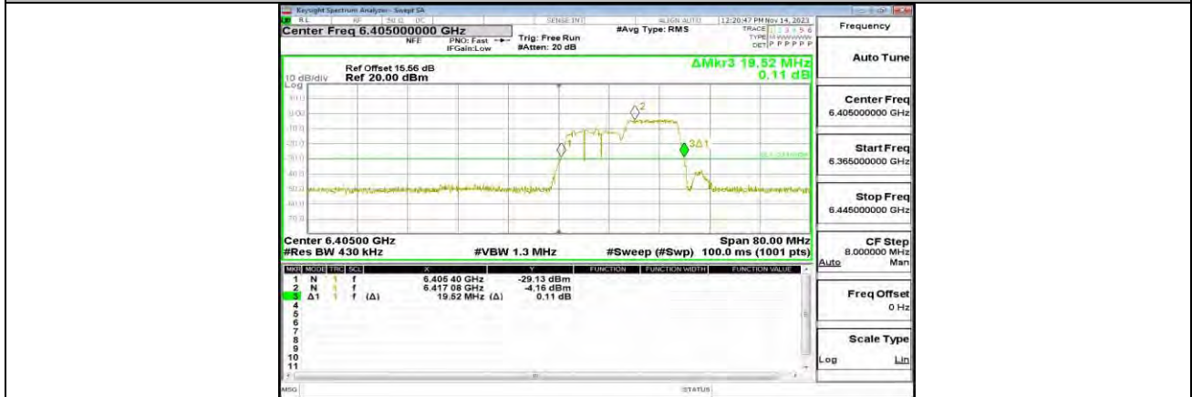
11AX40MIMO_ANT0_6405_106Tone_RU54
