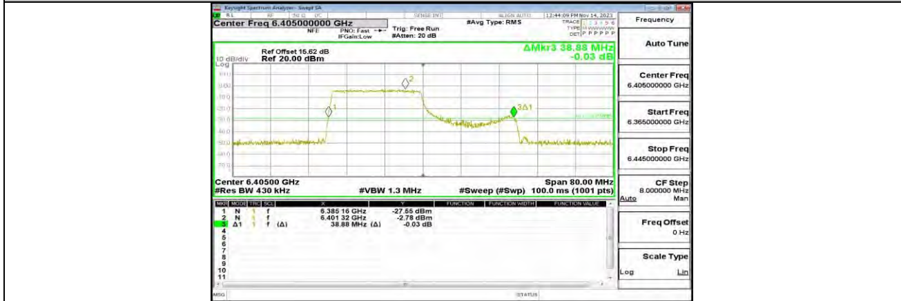
11AX40MIMO_ANT1_6405_242Tone_RU61
