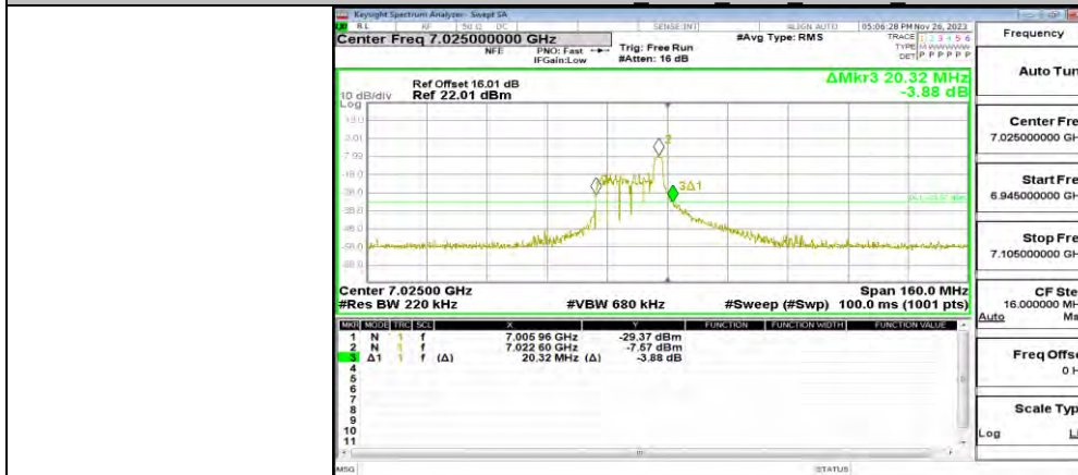
11AX80MIMO_ANT1_7025_26Tone_RU0
