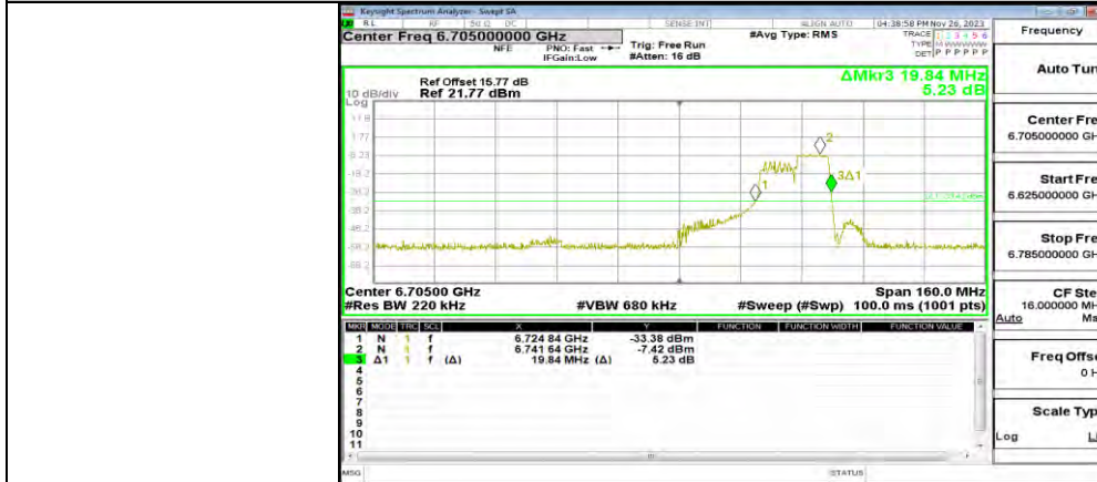
11AX80MIMO_ANT0_6705_106Tone_RU60
