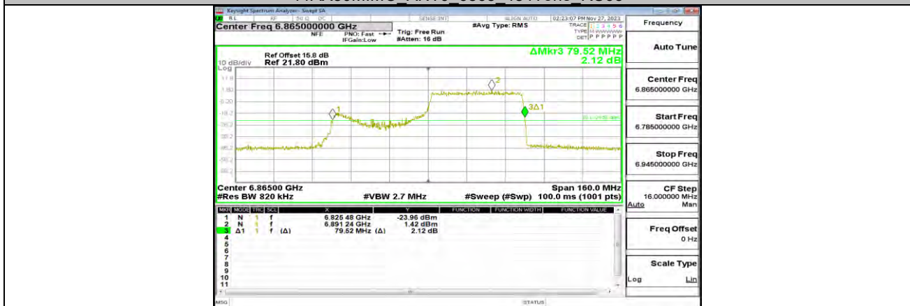
11AX80MIMO_ANT0_6865_484Tone_RU65
