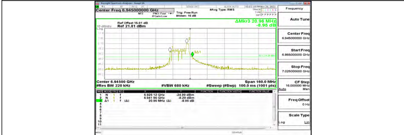
11AX80MIMO_ANT1_6945_26Tone_RU17
