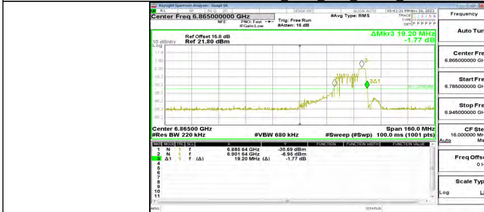
11AX80MIMO_ANT0_6865_52Tone_RU52
