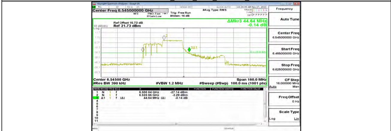
11AX80MIMO_ANT0_6545_242Tone_RU62
