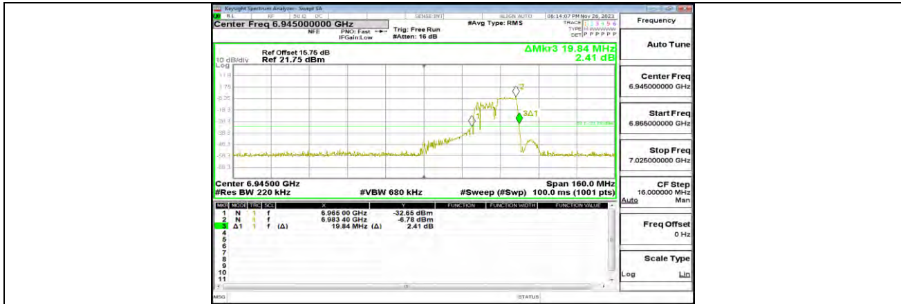
11AX80MIMO_ANT0_6945_106Tone_RU60
