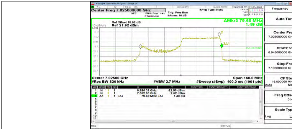
11AX80MIMO_ANT0_7025_484Tone_RU66
