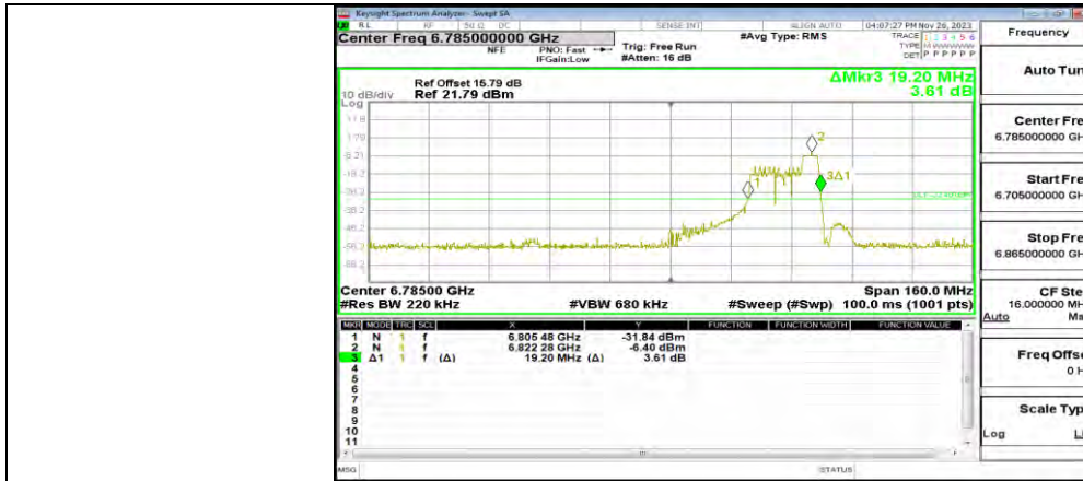
11AX80MIMO_ANT0_6785_52Tone_RU52
