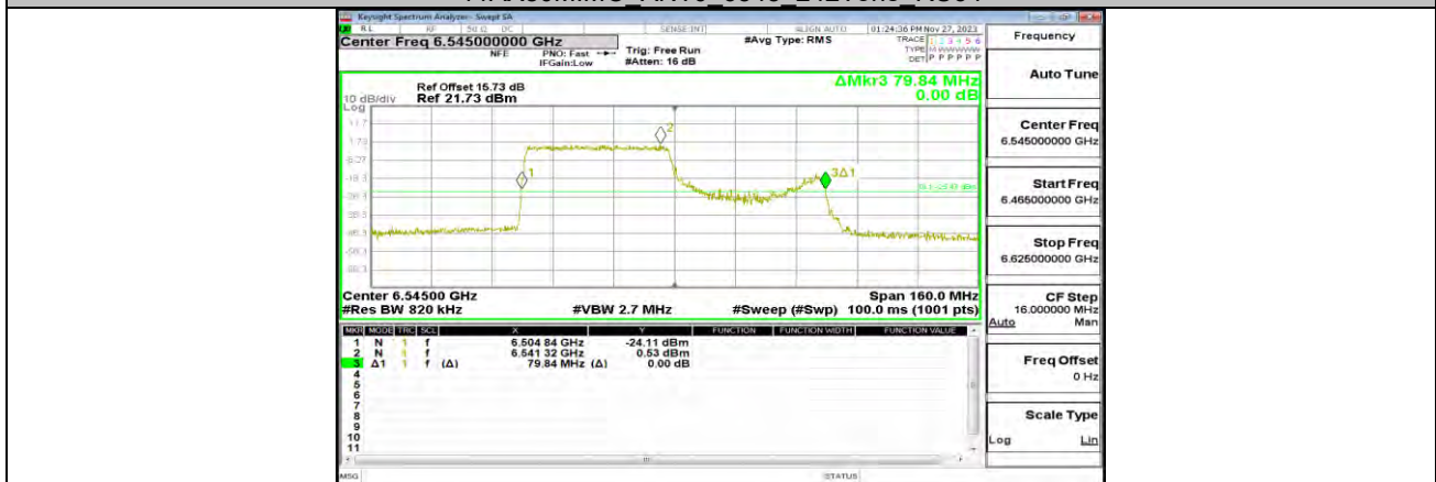
11AX80MIMO_ANT0_6545_242Tone_RU64
