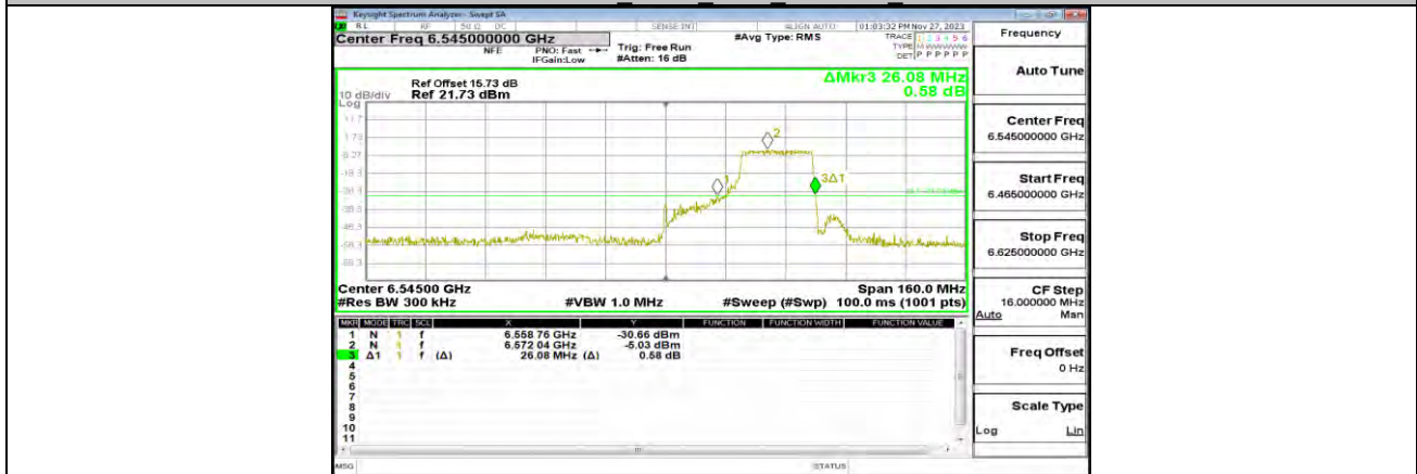
11AX80MIMO_ANT0_6545_242Tone_RU64
