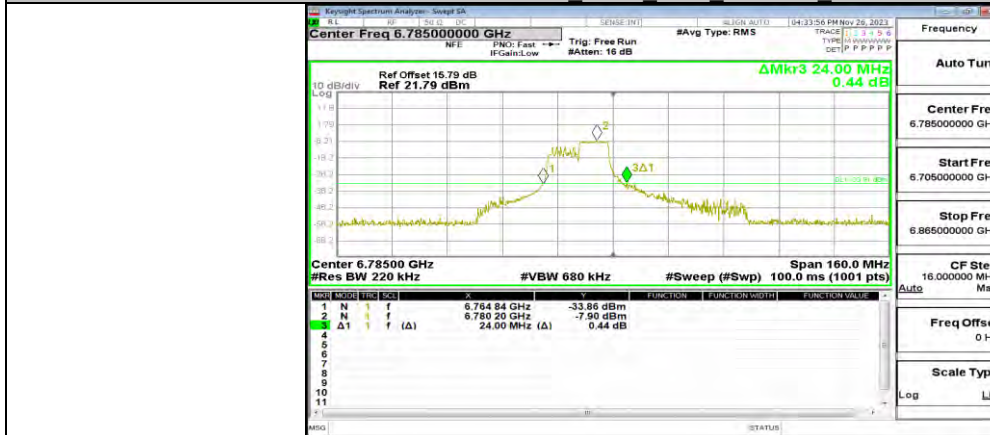
11AX80MIMO_ANT0_6785_106Tone_RU56
