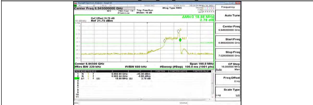
11AX80MIMO_ANT0_6945_26Tone_RU36
