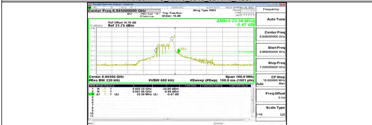
11AX80MIMO_ANT0_6945_52Tone_RU37
