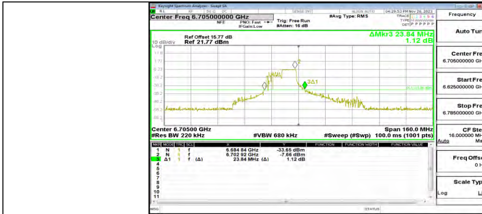
11AX80MIMO_ANT0_6705_106Tone_RU56
