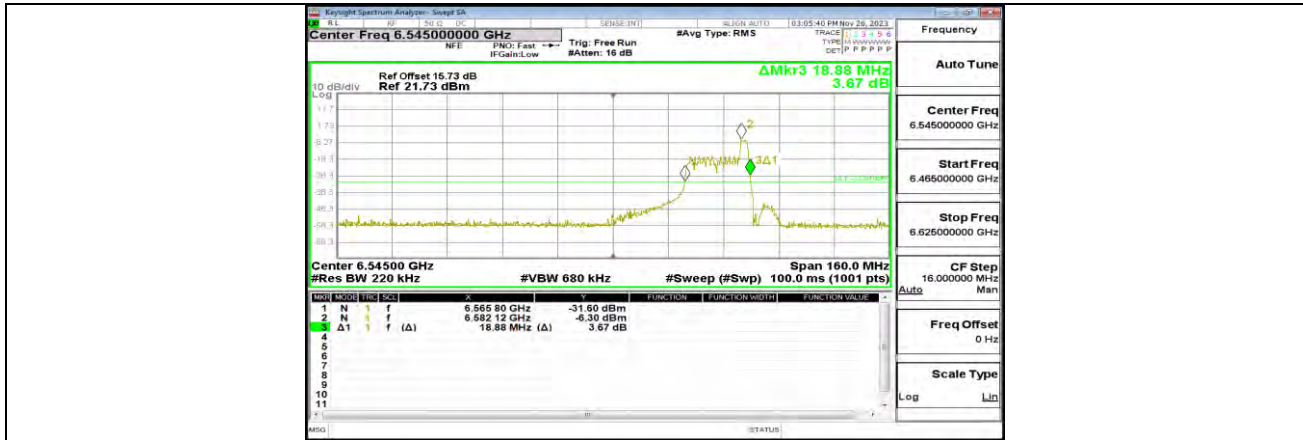
11AX80MIMO_ANT0_6545_26Tone_RU36
