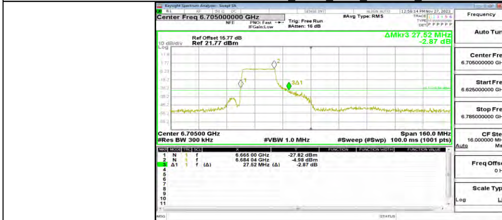
11AX80MIMO_ANT0_6705_242Tone_RU61
