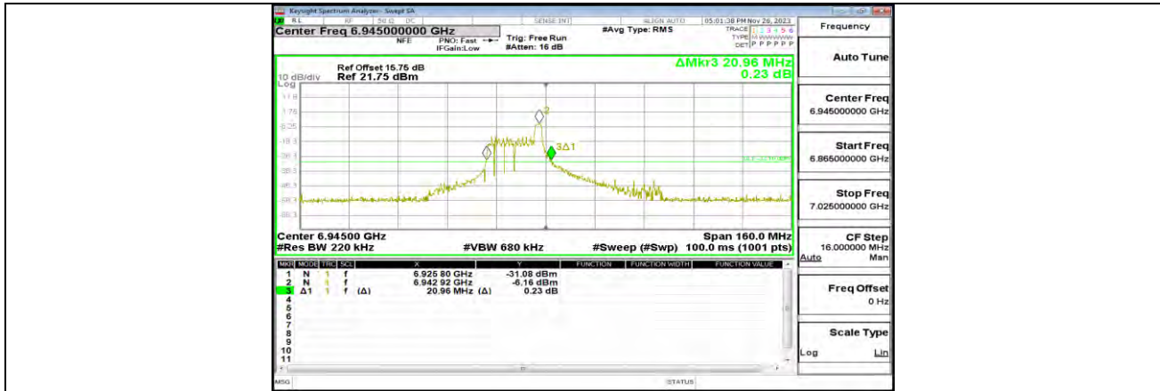
11AX80MIMO_ANT0_6945_26Tone_RU17
