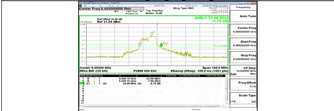
11AX80MIMO_ANT0_6465_106Tone_RU53
