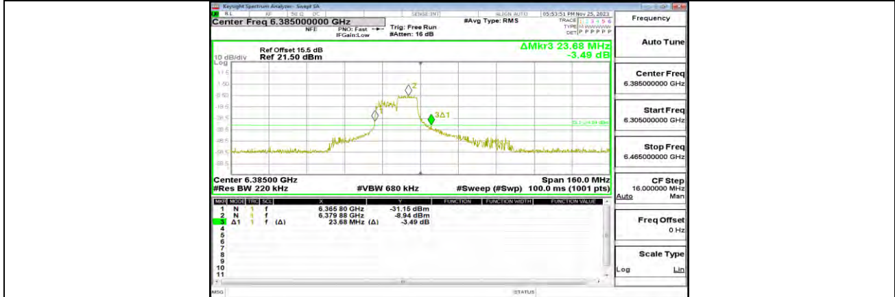
11AX80MIMO_ANT1_6385_106Tone_RU56
