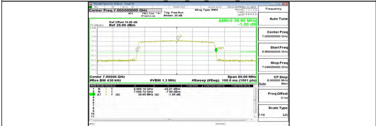
11AX40MIMO_ANT0_7005_484Tone_RU65
