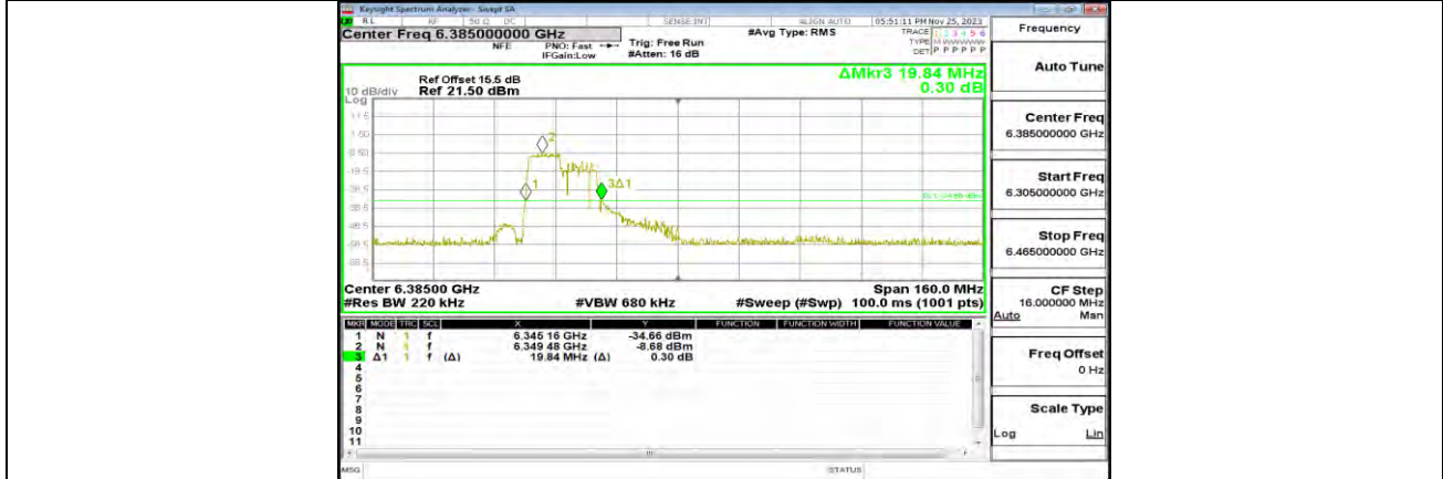
11AX80MIMO_ANT1_6385_106Tone_RU53
