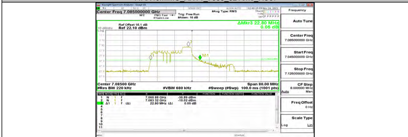
11AX40MIMO_ANT1_7085_52Tone_RU37
