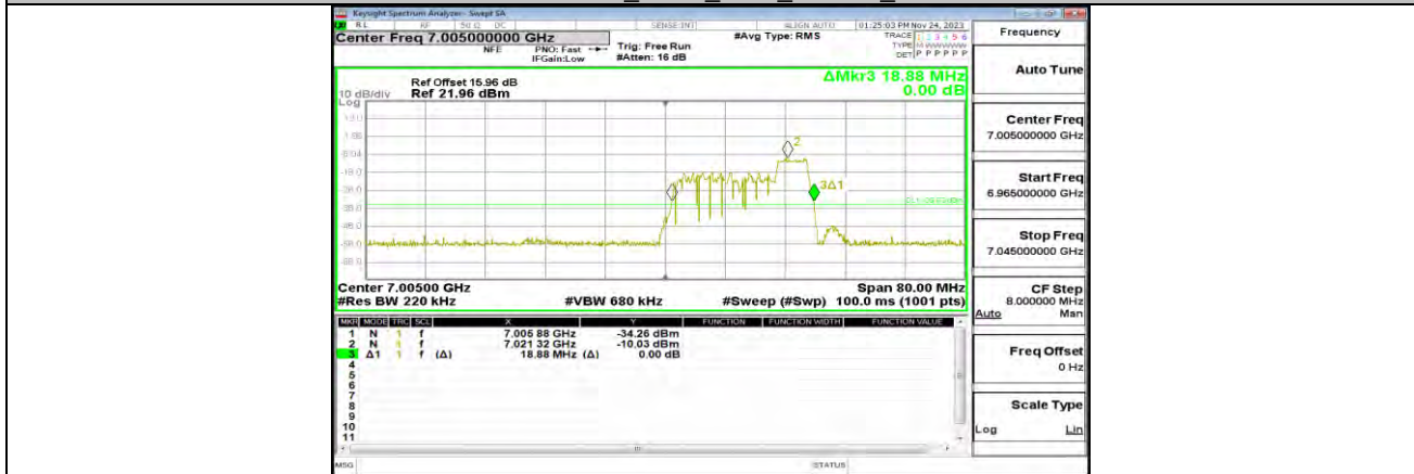
11AX40MIMO_ANT1_7005_52Tone_RU44
