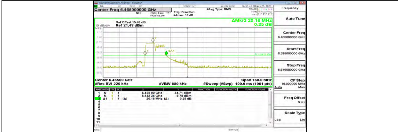
11AX80MIMO_ANT0_6465_106Tone_RU53
