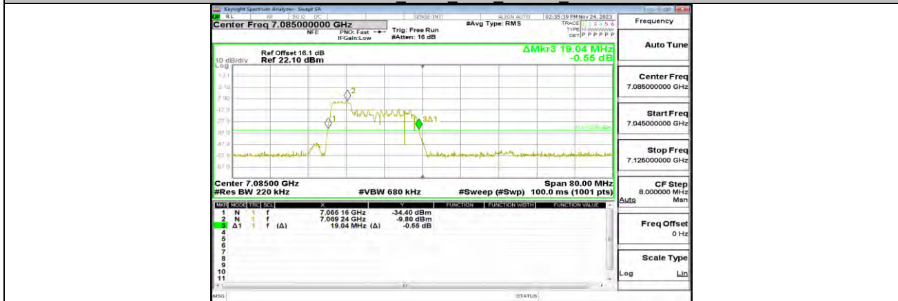
11AX40MIMO_ANT1_7085_52Tone_RU37
