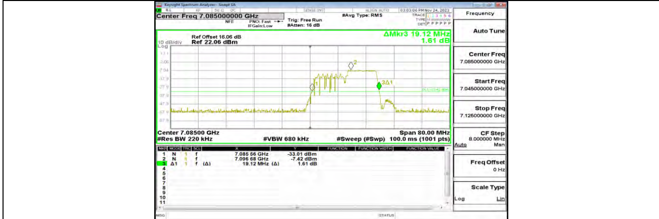
11AX40MIMO_ANT0_7085_106Tone_RU56
