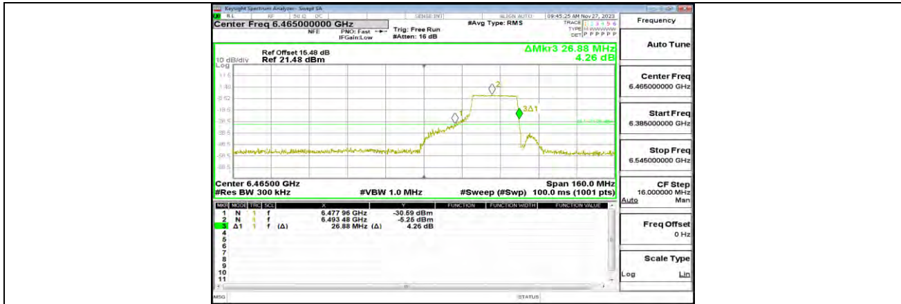
11AX80MIMO_ANT0_6465_242Tone_RU64
