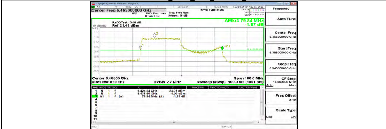
11AX80MIMO_ANT0_6465_484Tone_RU65
