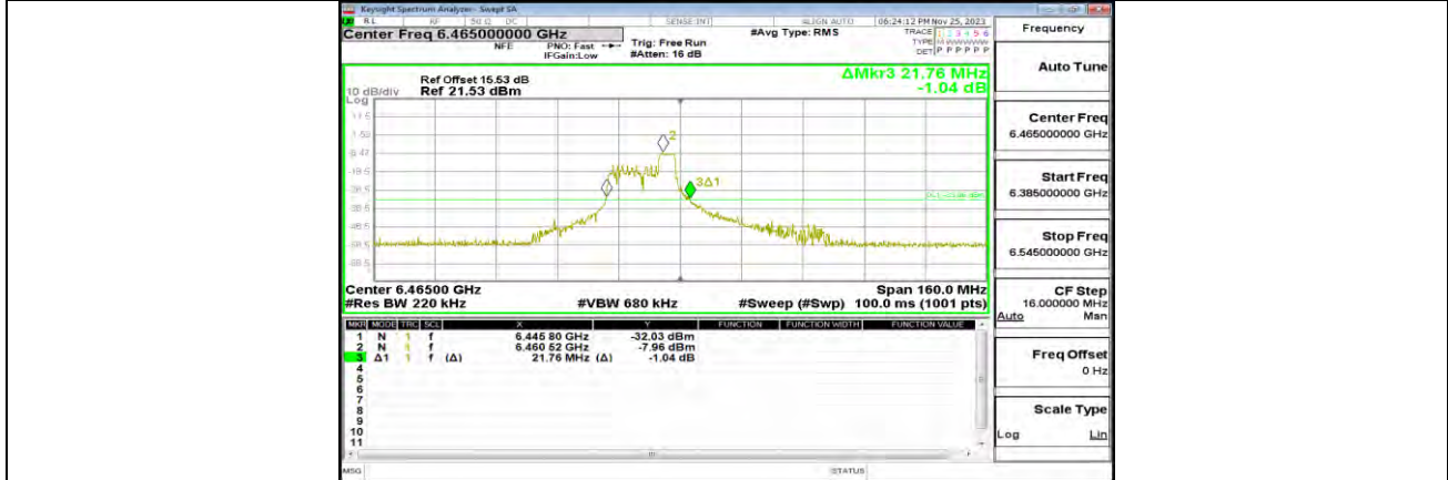
11AX80MIMO_ANT1_6465_52Tone_RU44
