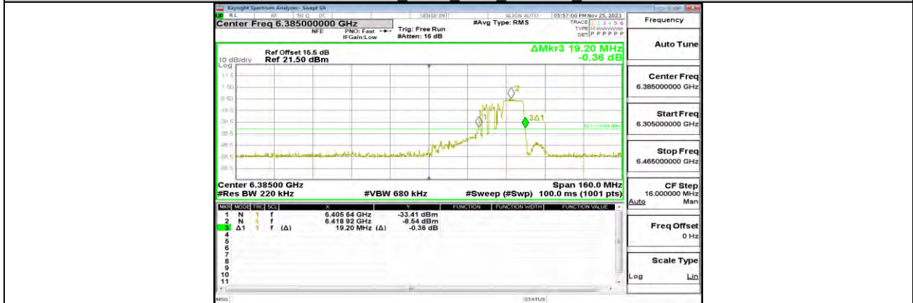
11AX80MIMO_ANT1_6385_106Tone_RU56
