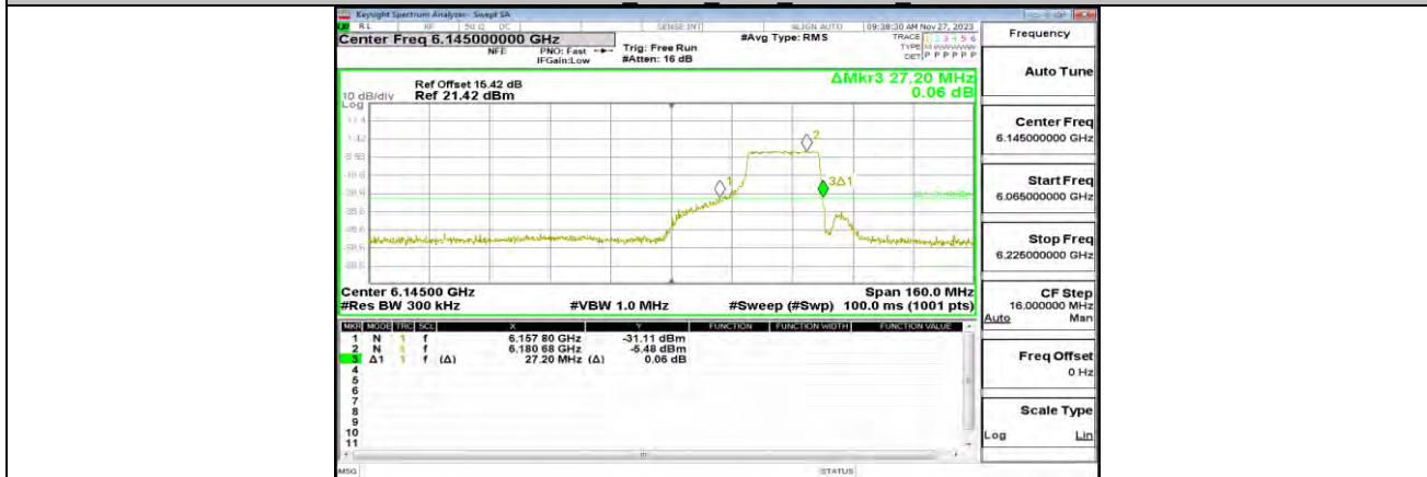
11AX80MIMO_ANT0_6145_242Tone_RU62
