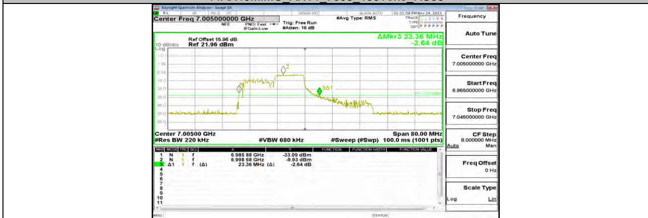
11AX40MIMO_ANT1_7005_106Tone_RU53
