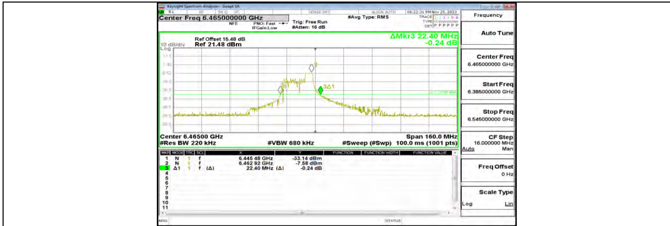
11AX80MIMO_ANT0_6465_52Tone_RU44
