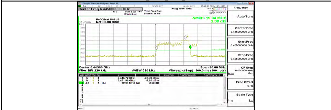
11AX40MIMO_ANT0_6445_52Tone_RU40
