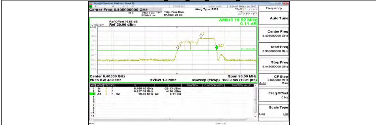
11AX40MIMO_ANT0_6405_106Tone_RU54
