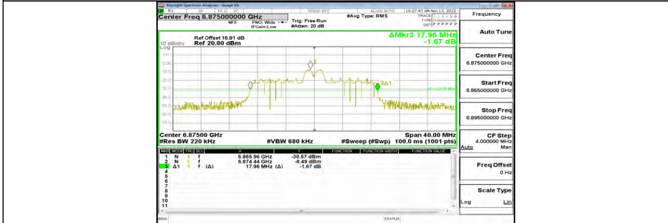
11AX20MIMO ANT1 6875 26Tone RU4
