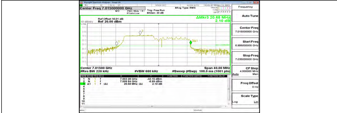
11AX20MIMO ANT1 7015 52Tone RU40
