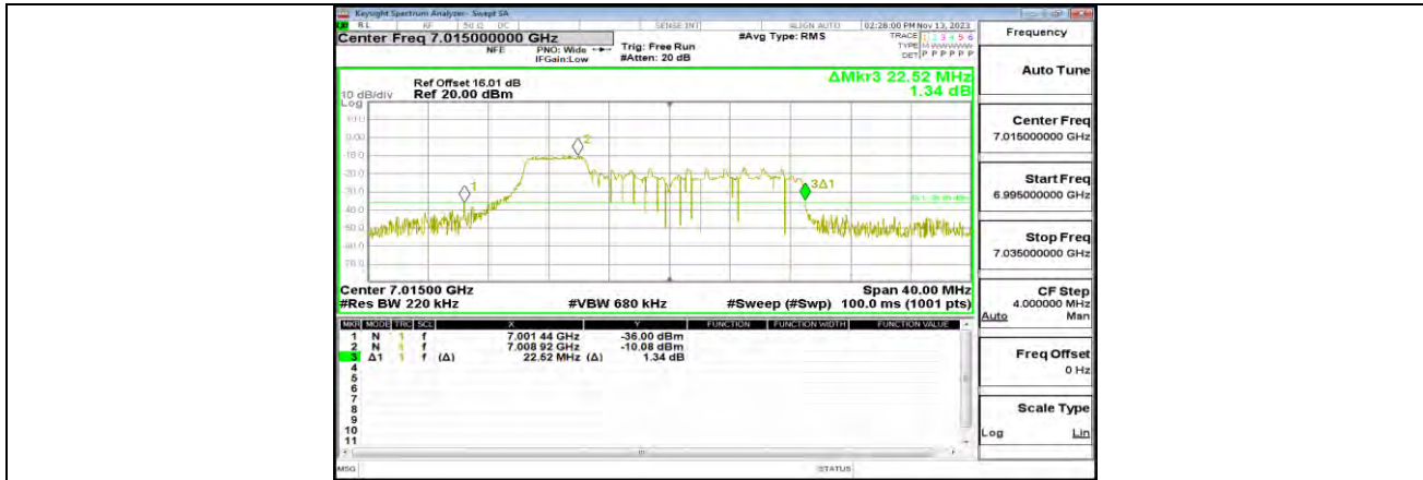
11AX20MIMO_ANT1_7015_52Tone_RU37
