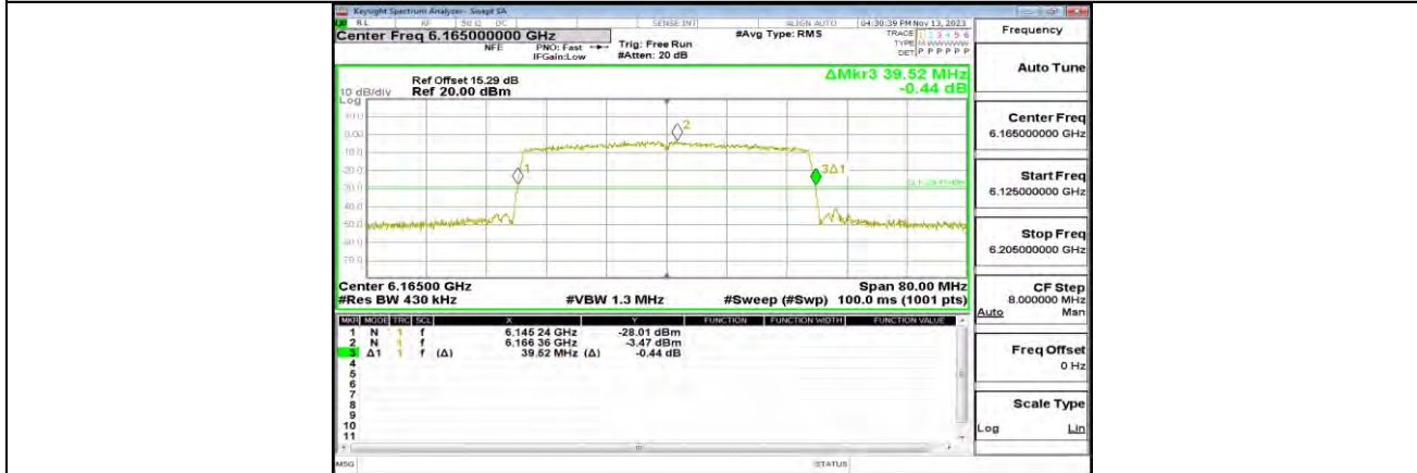
11AX40MIMO ANT1 6165 484Tone RU65
