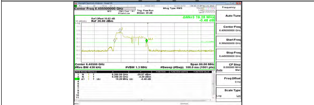
11AX40MIMO ANT1 6405 26Tone RU17
