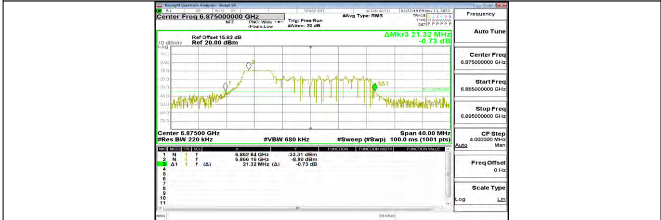
11AX20MIMO_ANT0_6875_52Tone_RU37
