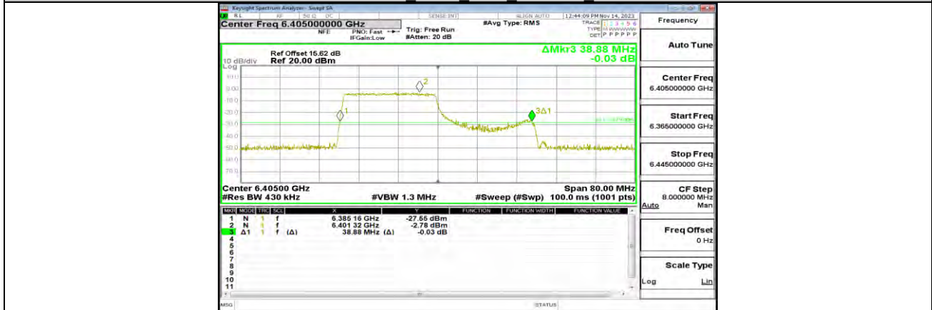
11AX40MIMO ANT1 6405 242Tone RU61
