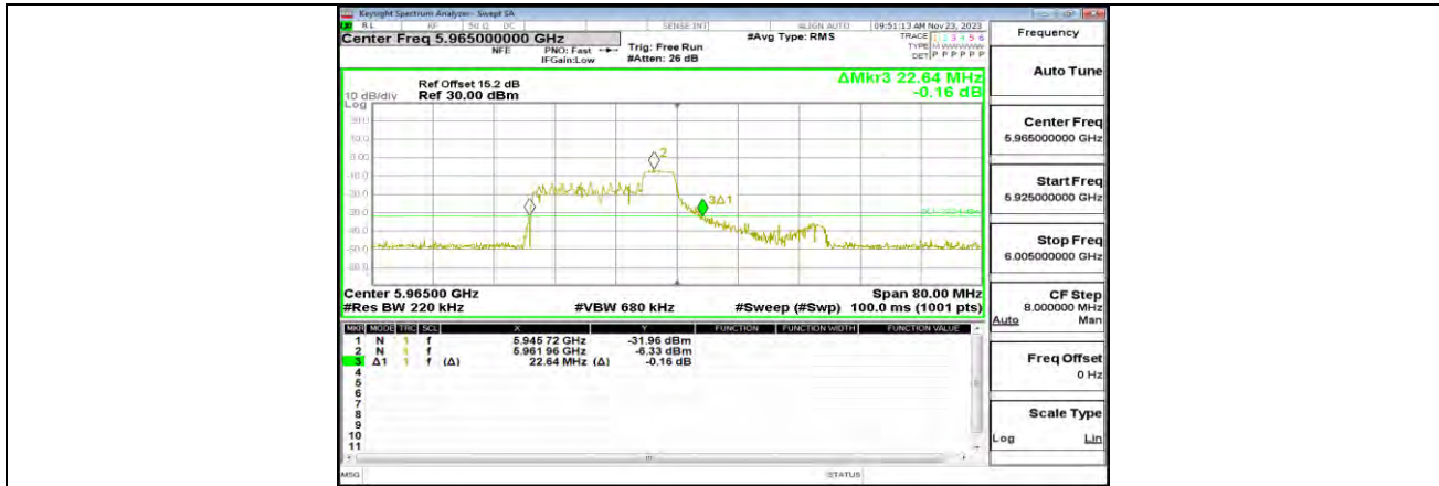
11AX40MIMO_ANT0_5965_52Tone_RU40
