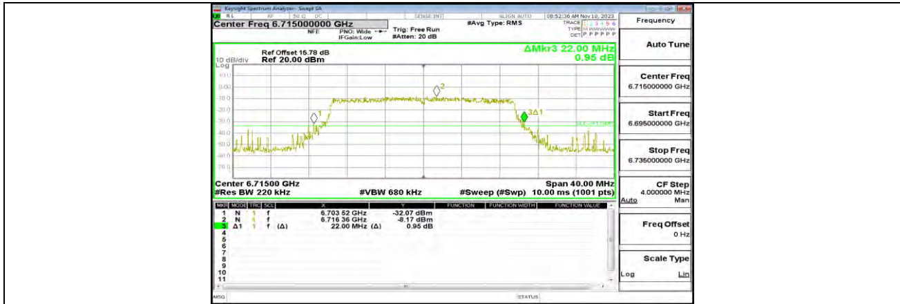
11AX20MIMO ANT1 6715 242Tone RU61
