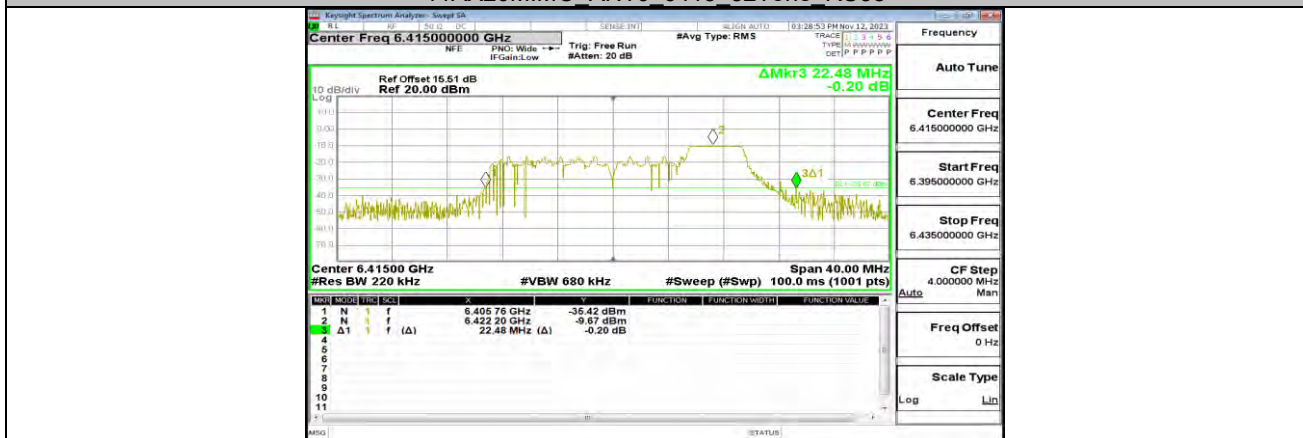
11AX20MIMO_ANT0_6415_52Tone_RU38
