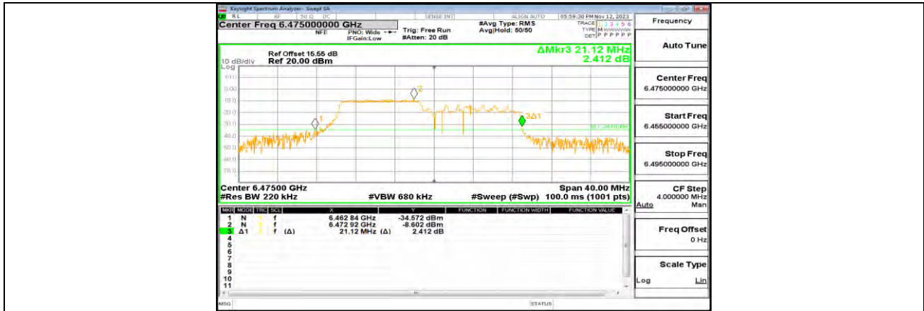
11AX20MIMO ANT1 6475 106Tone RU53
