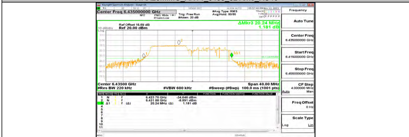
11AX20MIMO ANT1 6435 52Tone RU40
