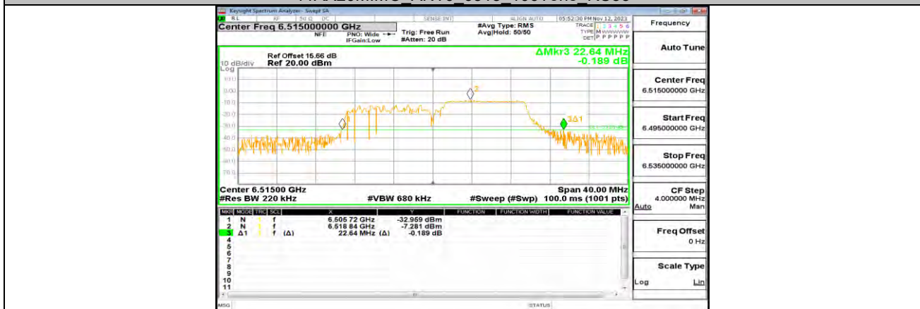
11AX20MIMO_ANT0_6515_106Tone_RU53
