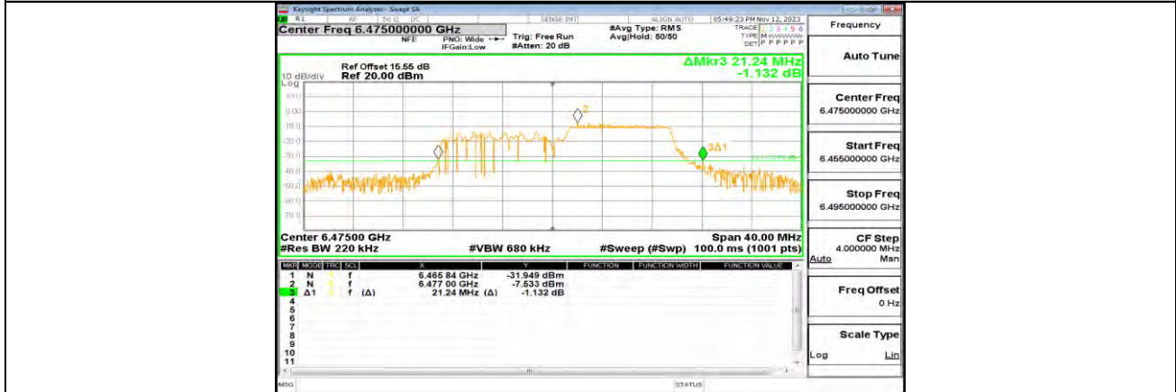
11AX20MIMO ANT1 6475 106Tone RU54
