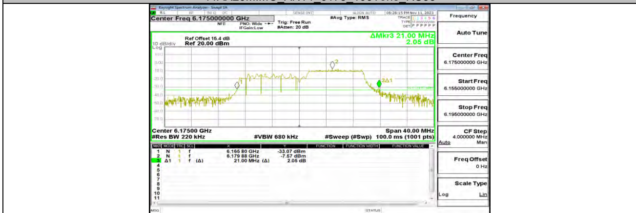
11AX20MIMO_ANT1_6175_106Tone_RU53
