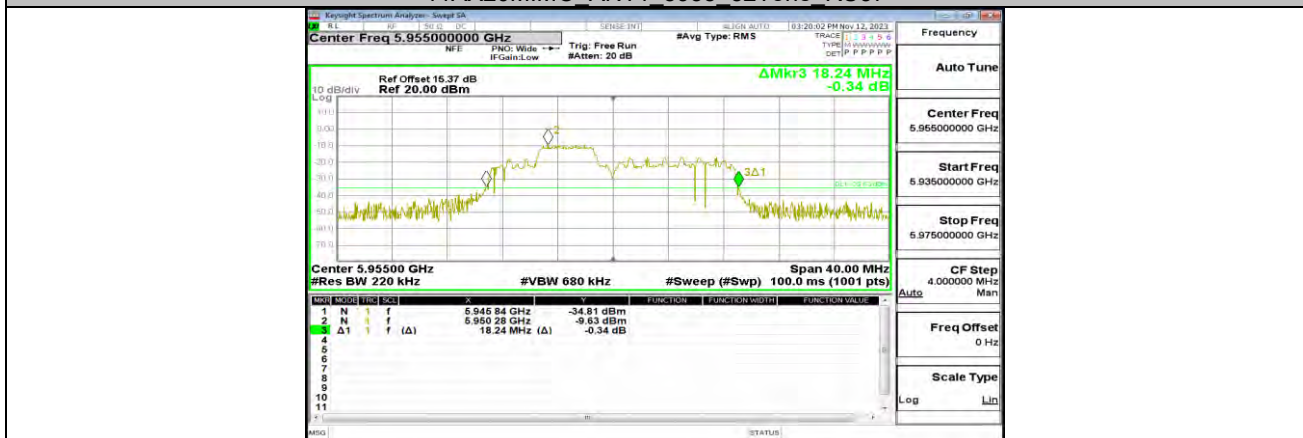
11AX20MIMO ANT1 5955 52Tone RU37
