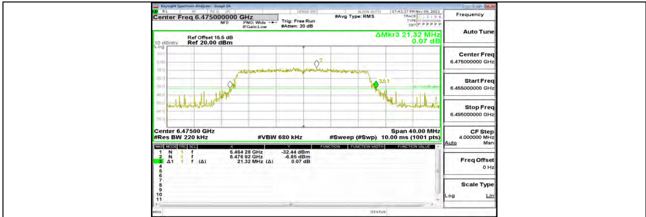
11AX20MIMO_ANT0_6475_242Tone_RU61
