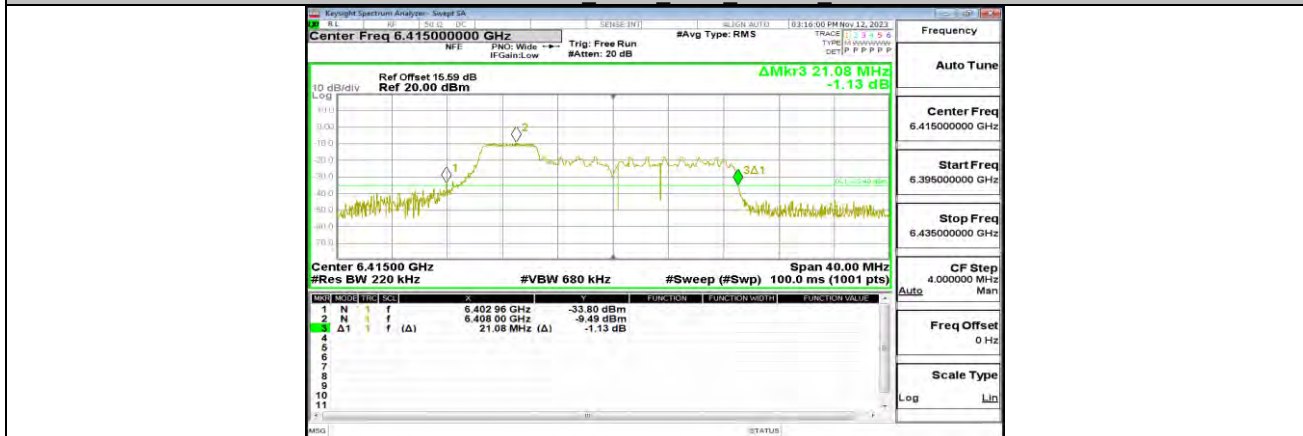
11AX20MIMO ANT1 6415 26Tone RU8
