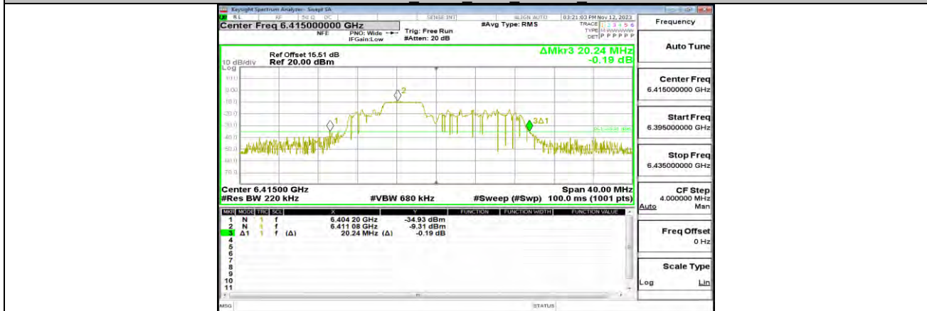
11AX20MIMO_ANT0_6415_52Tone_RU38
