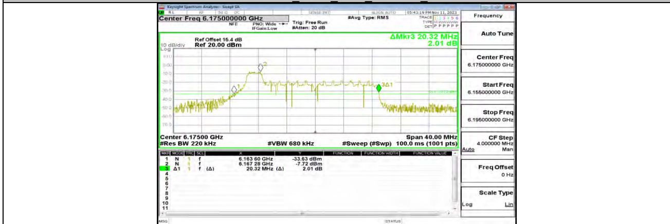
11AX20MIMO_ANT0_6175_242Tone_RU61
