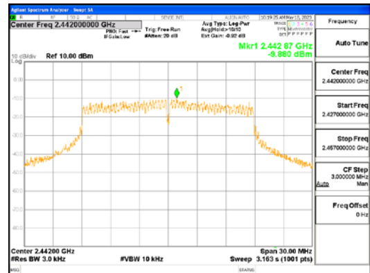
ANT L, 802.11n_HT20
