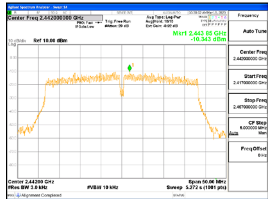
ANT L, 802.11n_HT40
