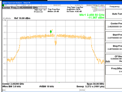
ANTI, 802.11n_HT40
